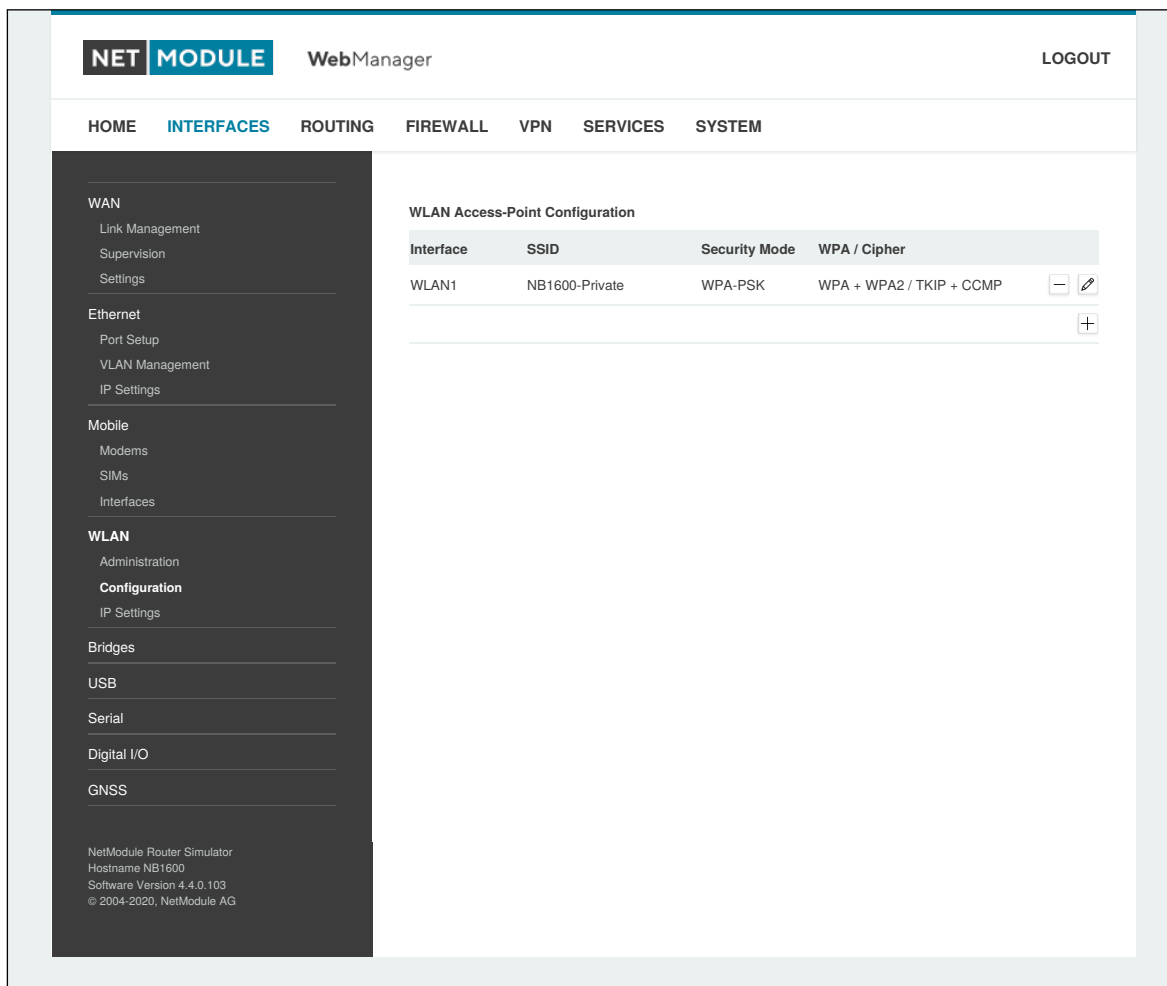
Abbildung 5.18.: WLAN-Konfiguration
