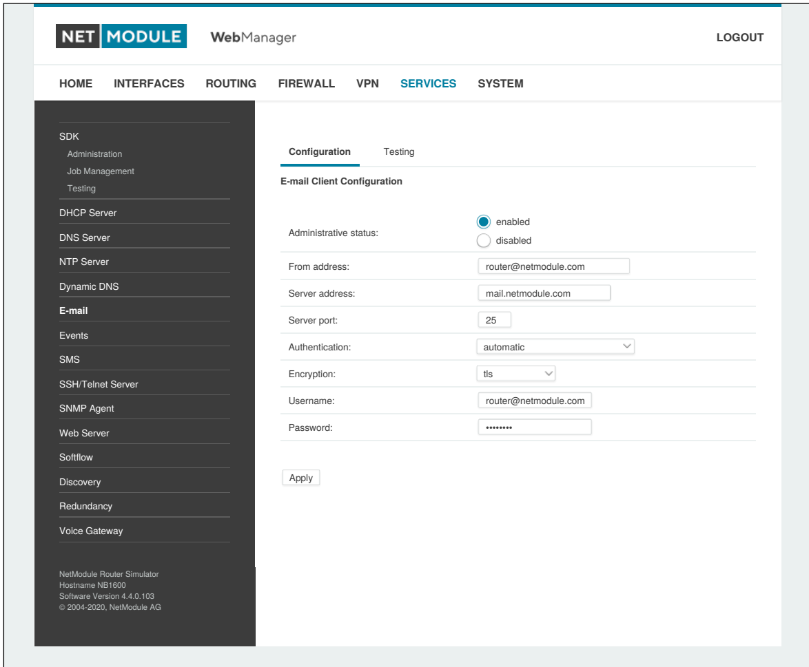
Abbildung 5.48.: E-Mail-Einstellungen
