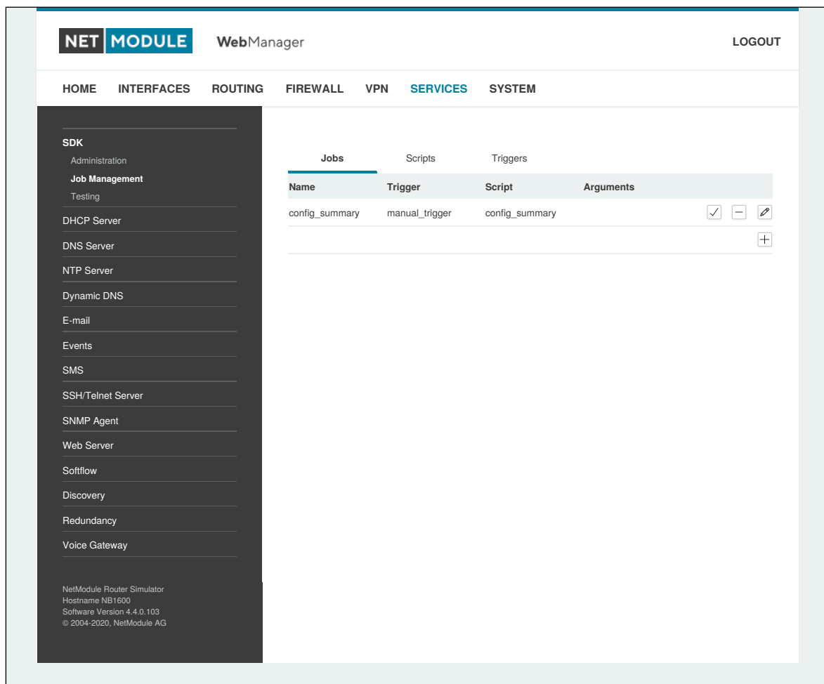
Abbildung 5.41.: SDK-Jobs
