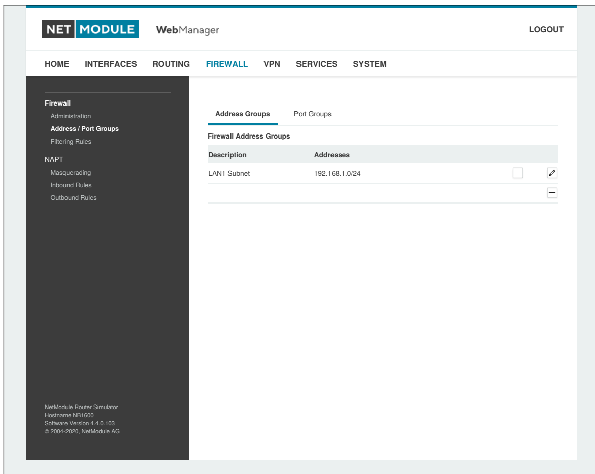
Abbildung 5.27.: Firewall-Gruppen
