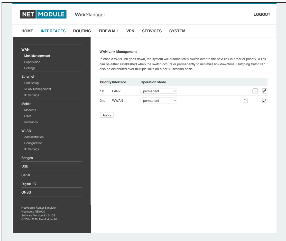
Abbildung 5.3.: WAN-Verbindungen
