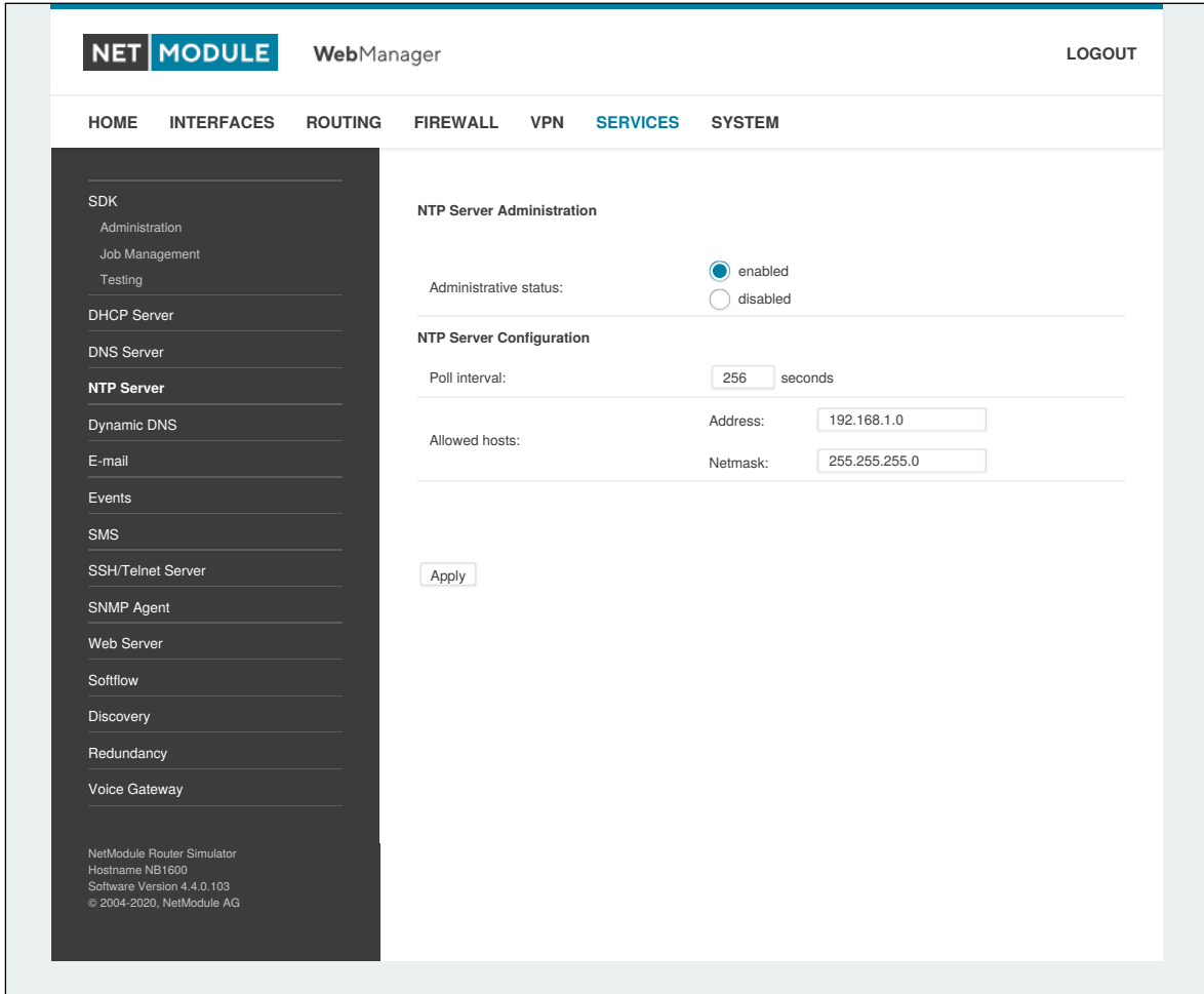
Abbildung 6.46.: NTP-Server
