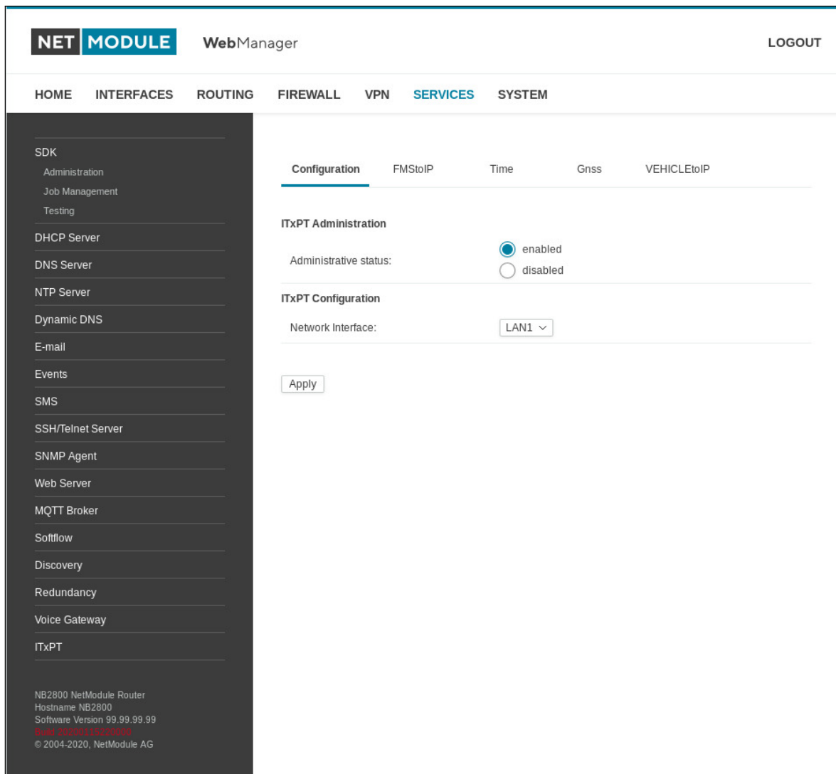
Abbildung 6.53.: ITxPT-Konfiguration
