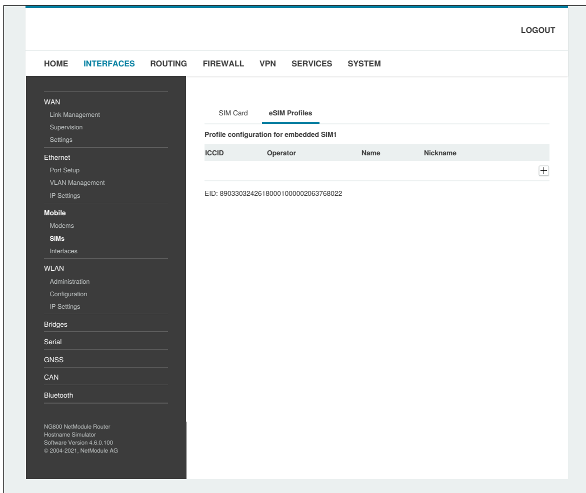
Abbildung 6.14.: eSIM-Profile
