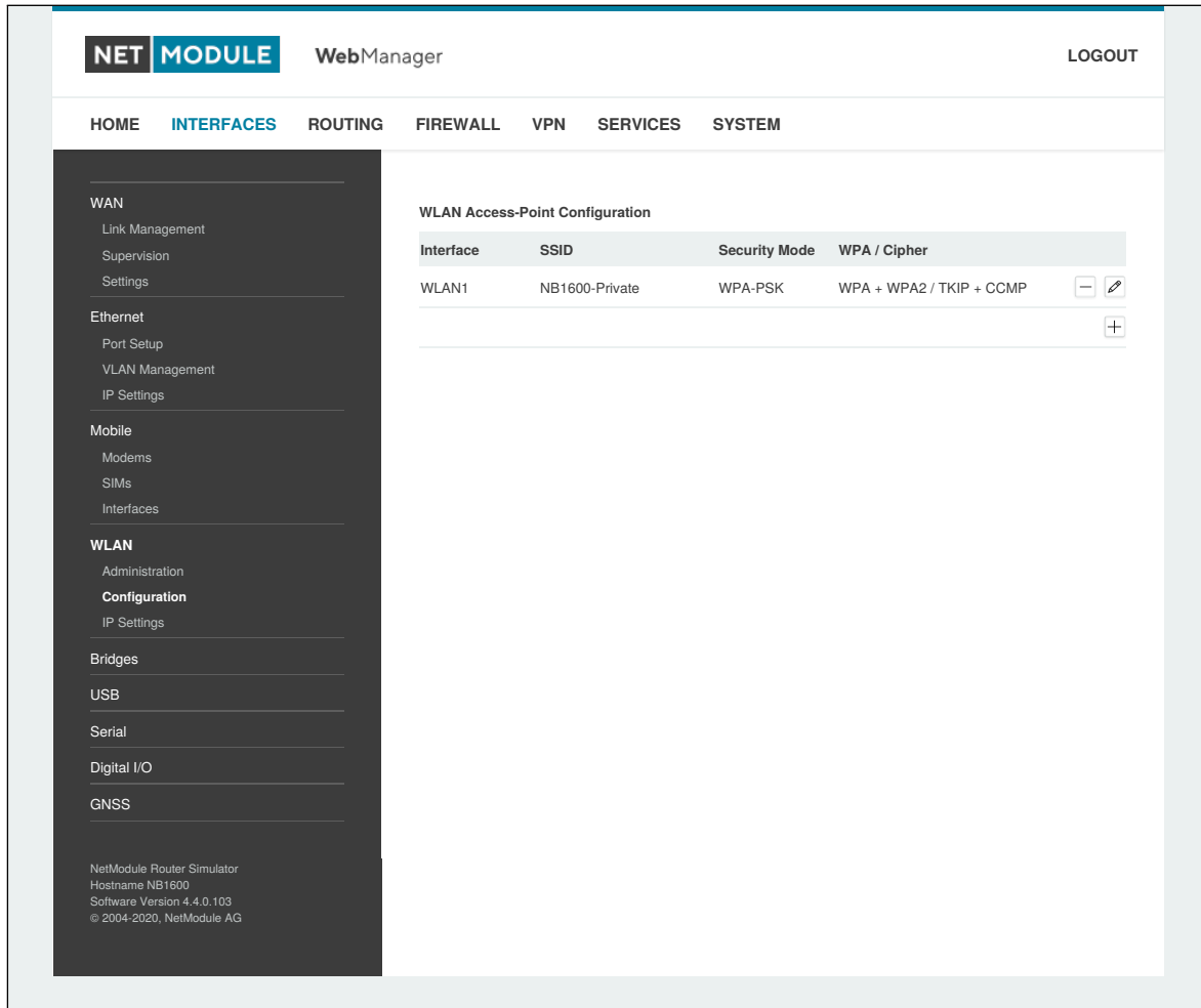
Abbildung 6.18.: WLAN-Konfiguration
