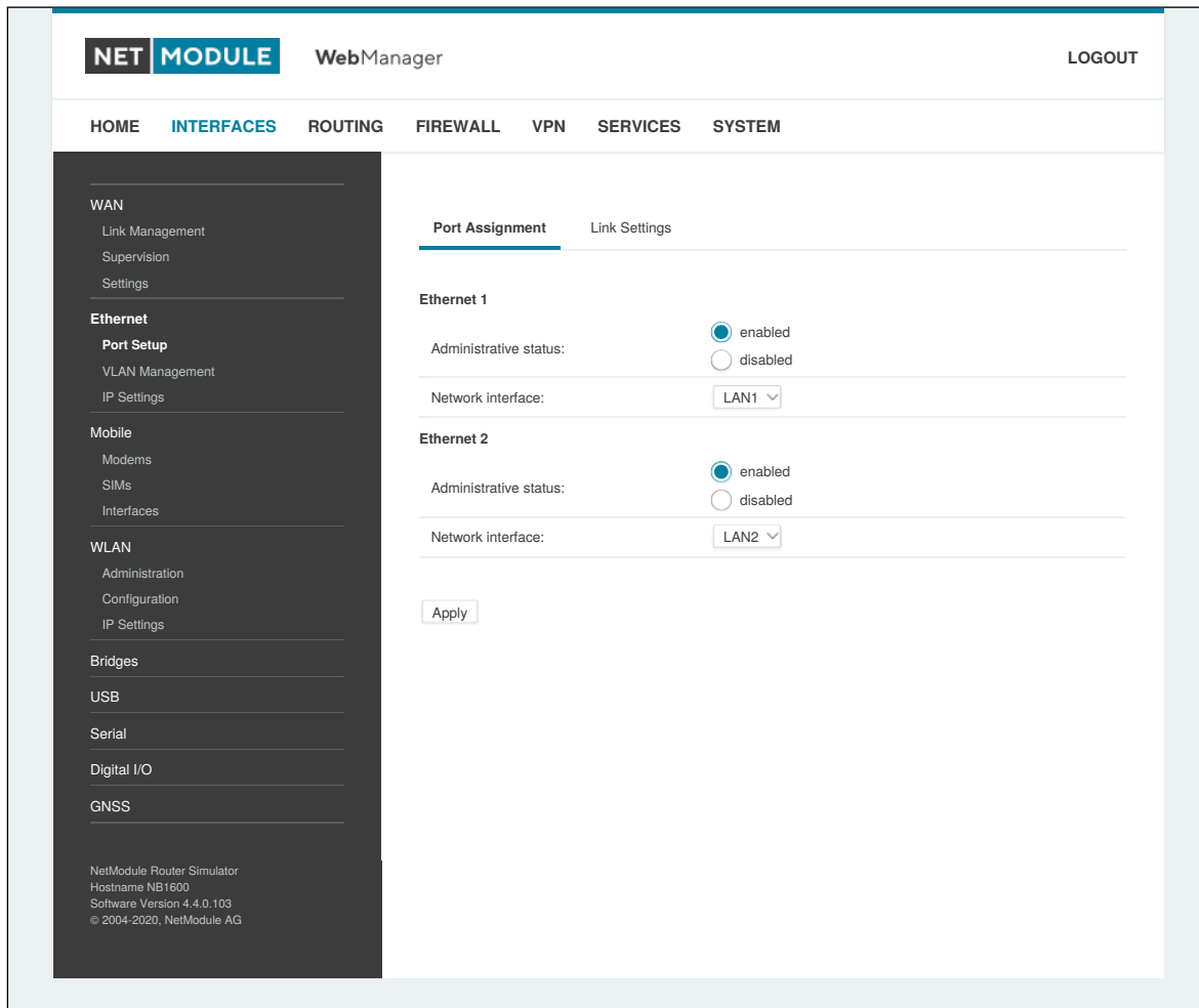
Abbildung 6.6.: Ethernet-Anschlüsse
