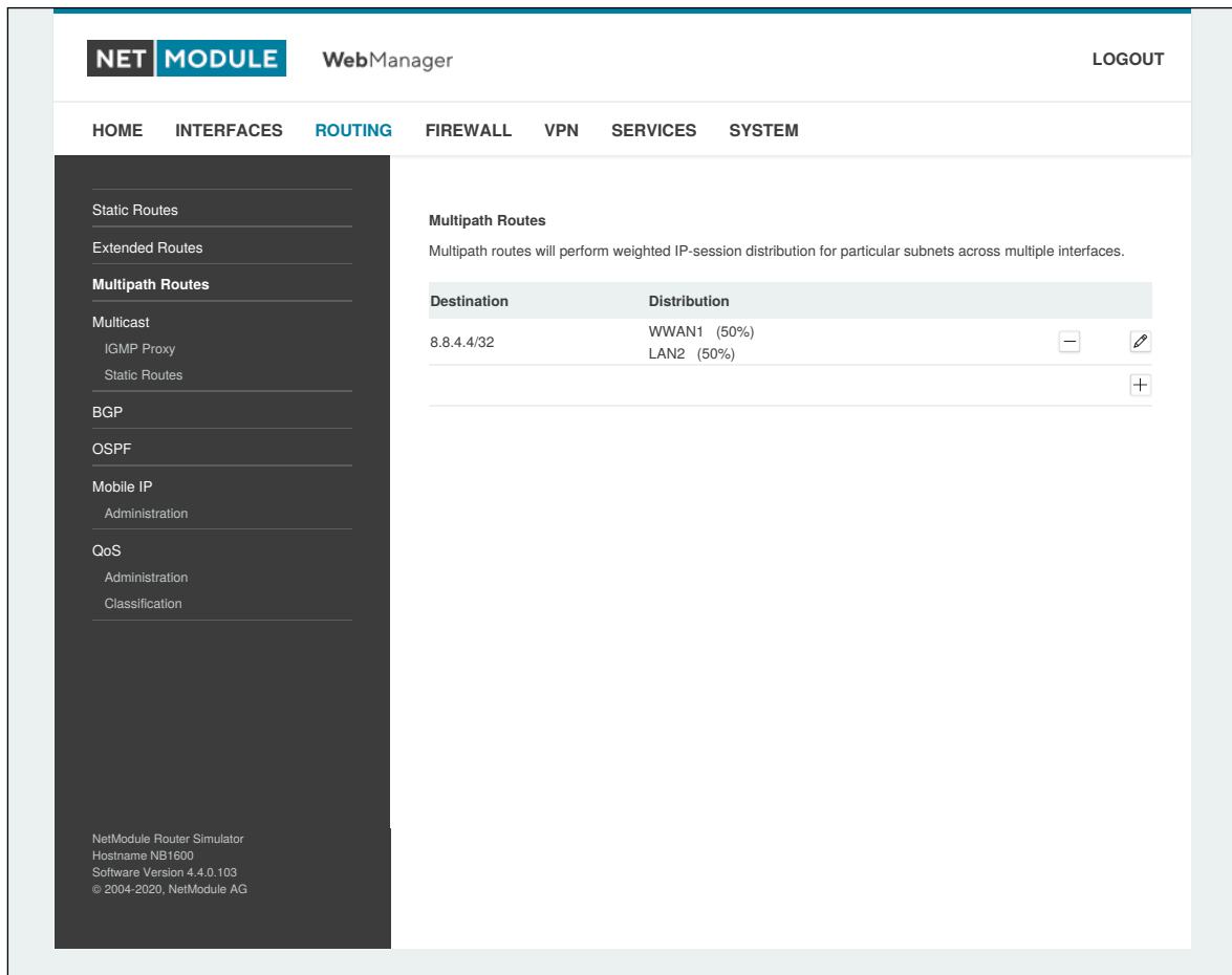
Abbildung 6.27.: Multipath-Routing
