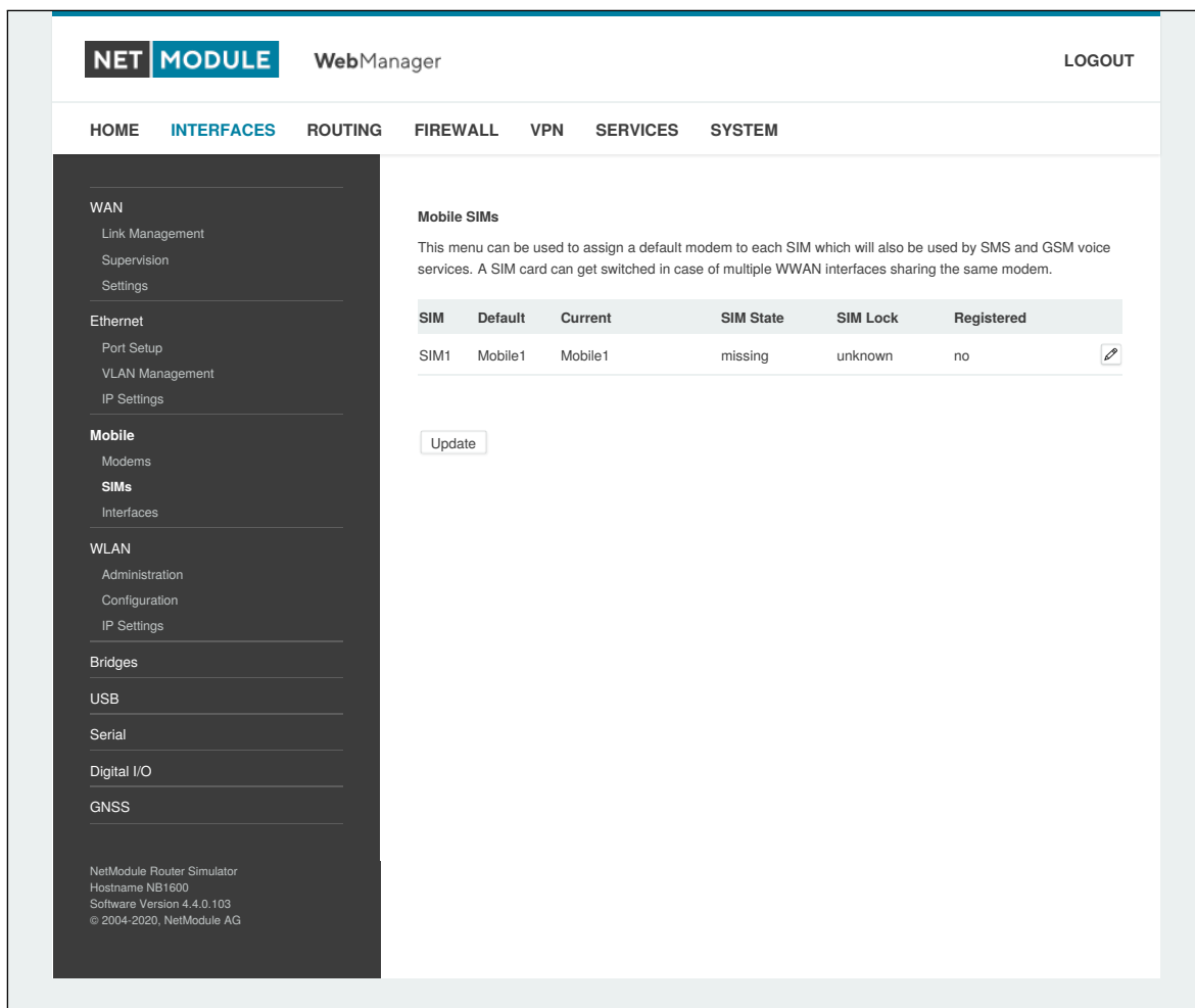
Abbildung 6.15.: SIM-Karten
