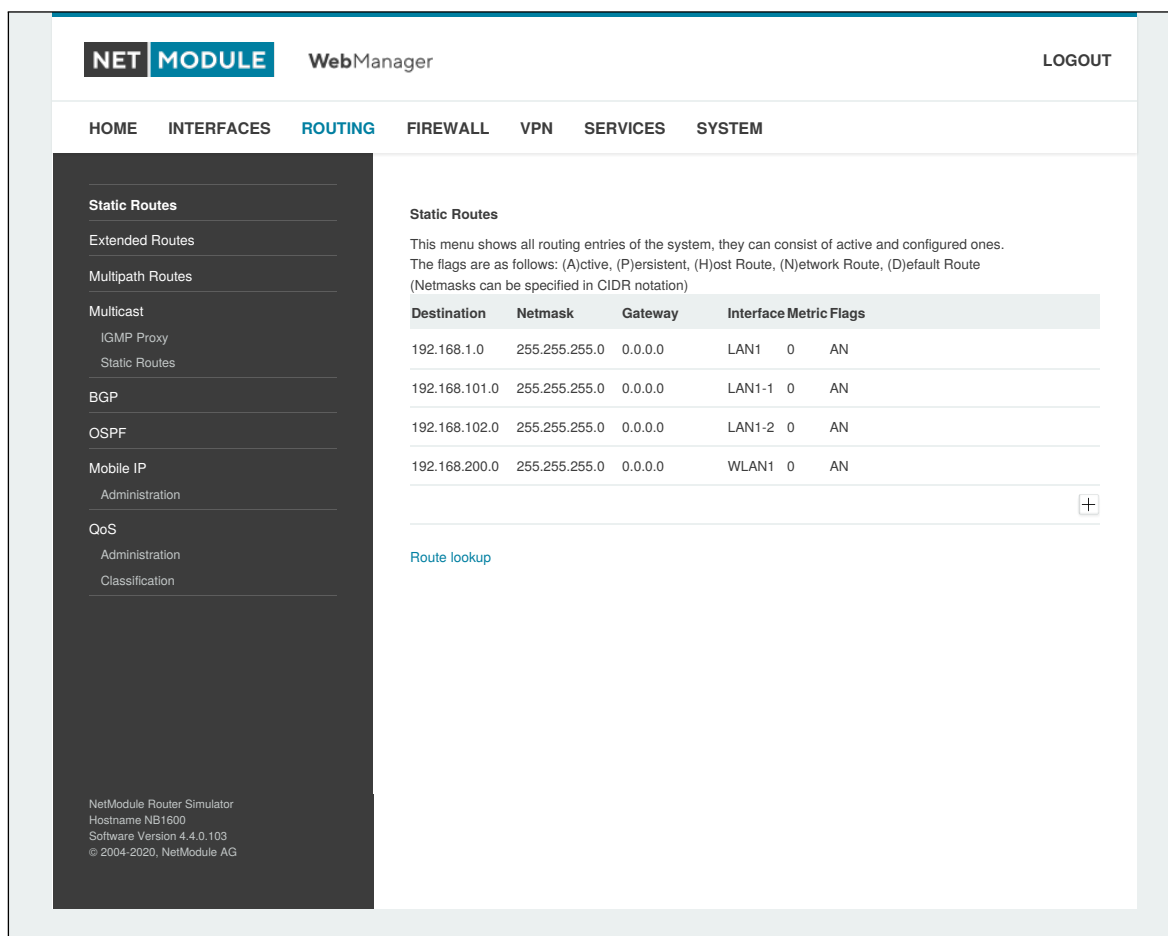
Abbildung 6.26.: Statisches Routing
