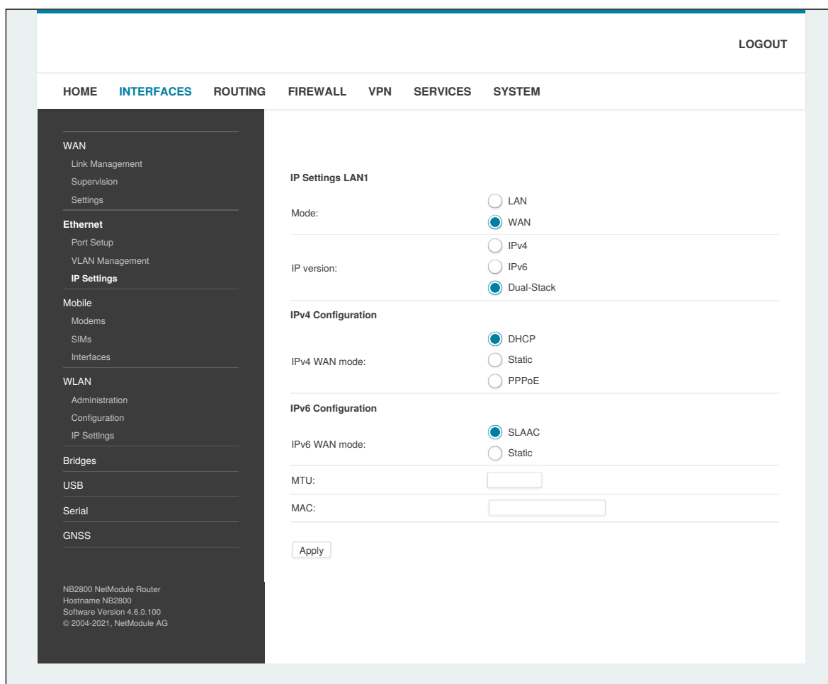
Abbildung 6.14.: IP Einstellungen - WAN Schnittstelle
