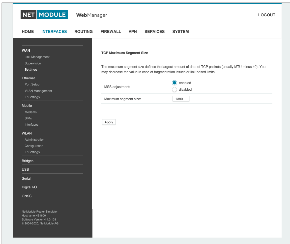
Abbildung 6.6.: WAN-Einstellungen
