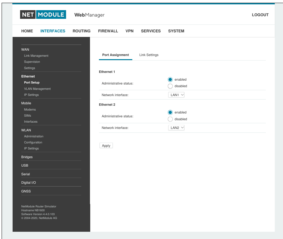
Abbildung 6.7.: Ethernet-Anschlüsse
