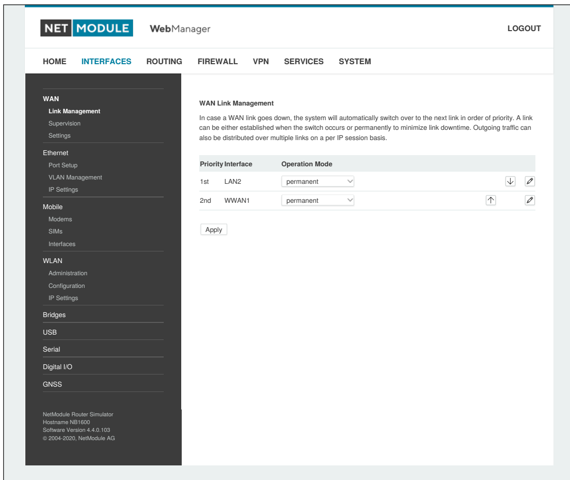
Abbildung 6.4.: WAN-Verbindungen
