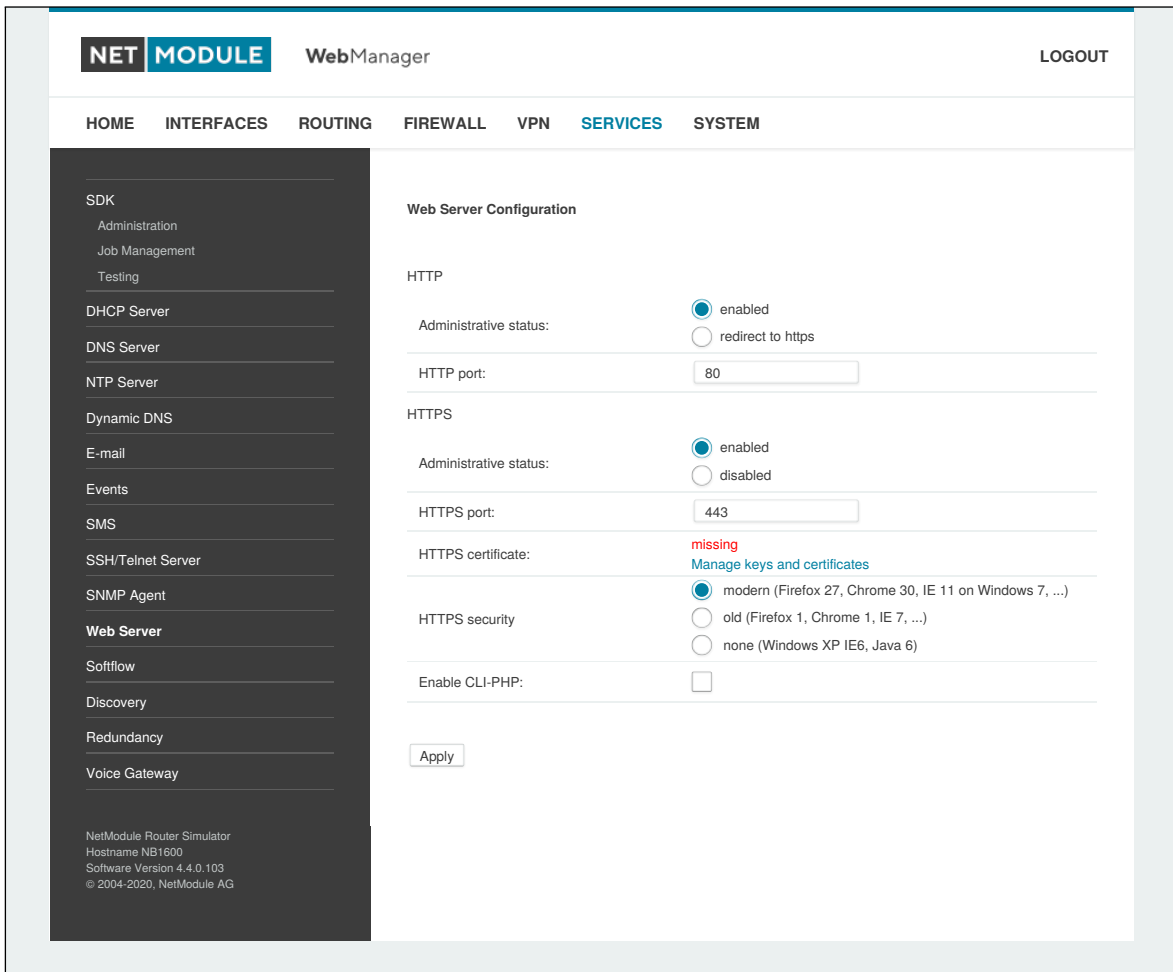
Abbildung 6.53.: Webserver
