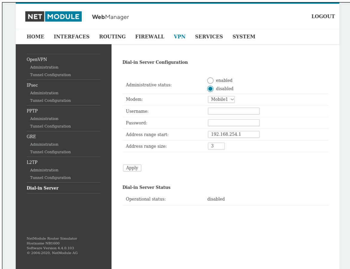
Abbildung 6.42.: Einwahlserver-Einstellungen
