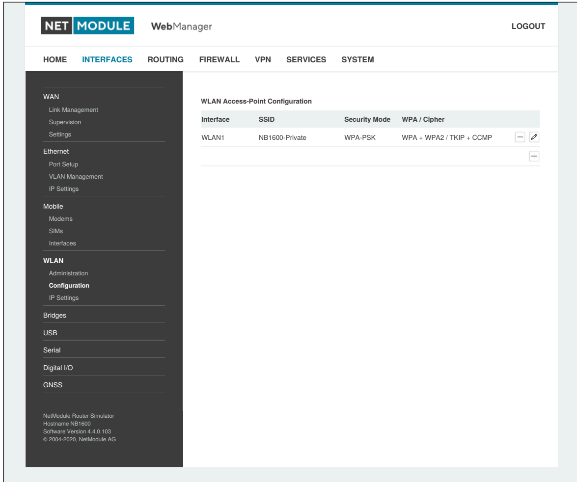
Abbildung 6.66.: WLAN administration
