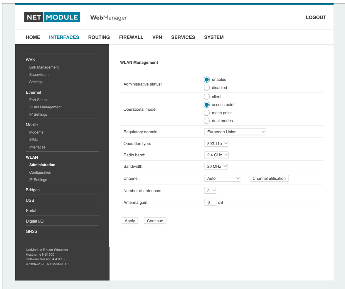
Abbildung 5.17.: WLAN-Verwaltung
