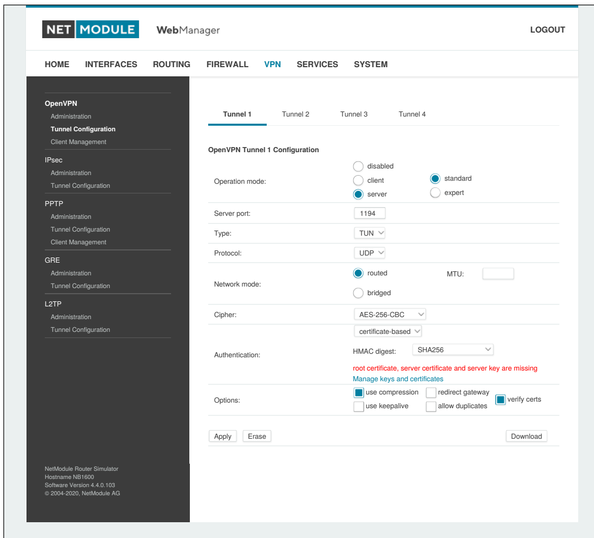
Abbildung 5.33.: Konfiguration von OpenVPN
