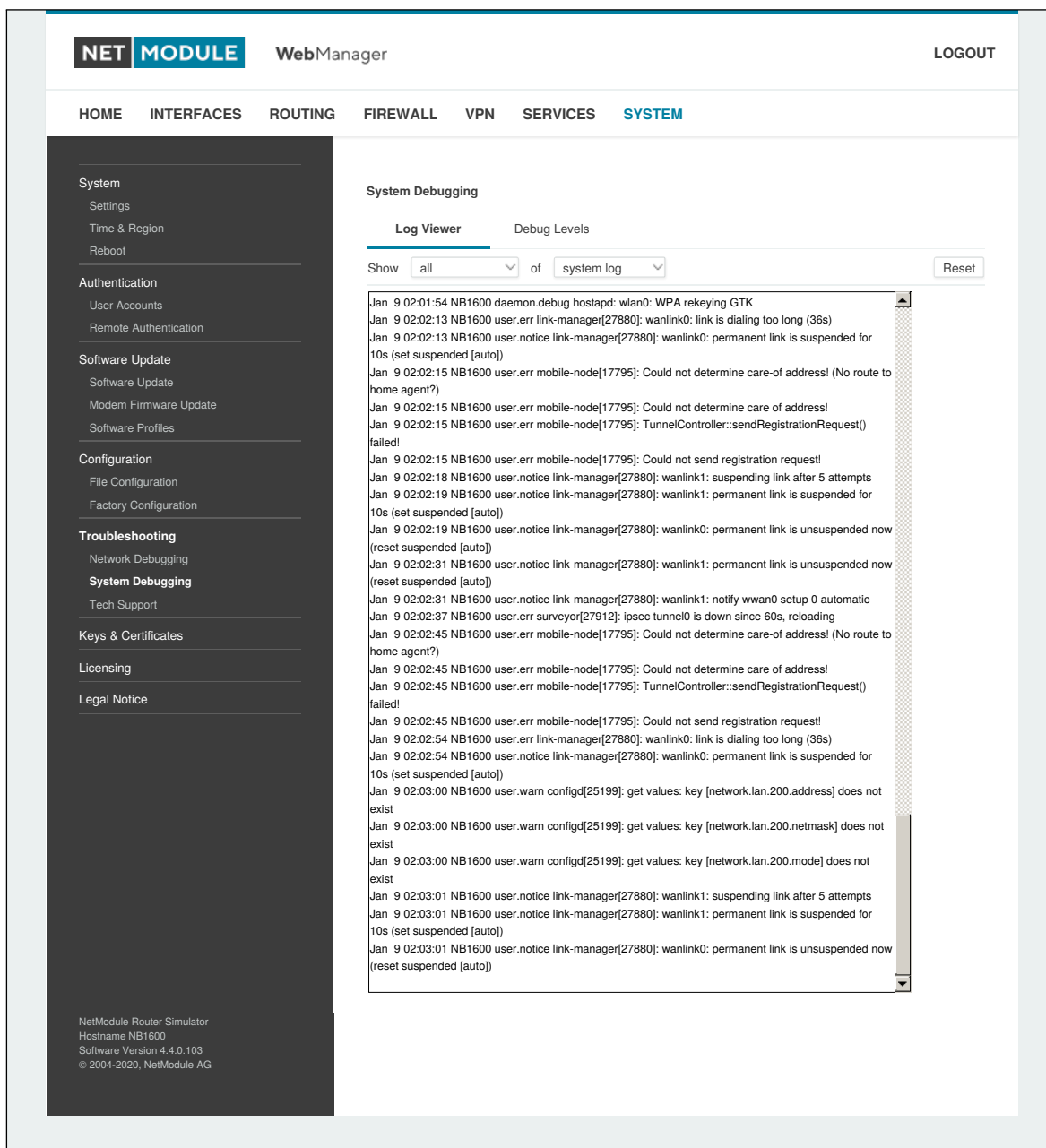
Abbildung 5.67.: Log-Viewer
