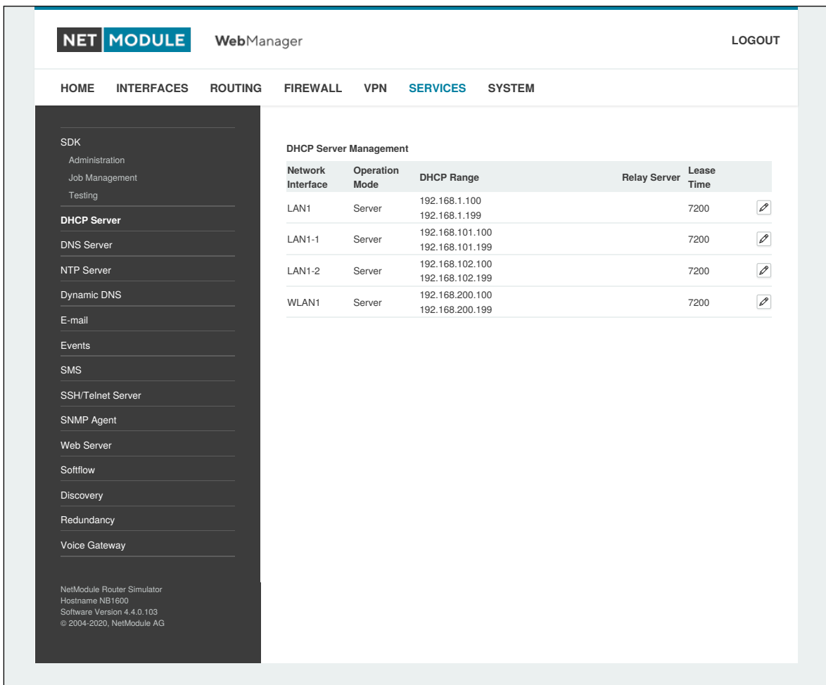
Abbildung 5.43.: DHCP-Server
