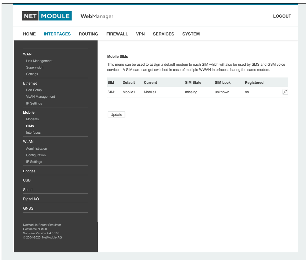
Abbildung 5.13.: SIM-Karten
