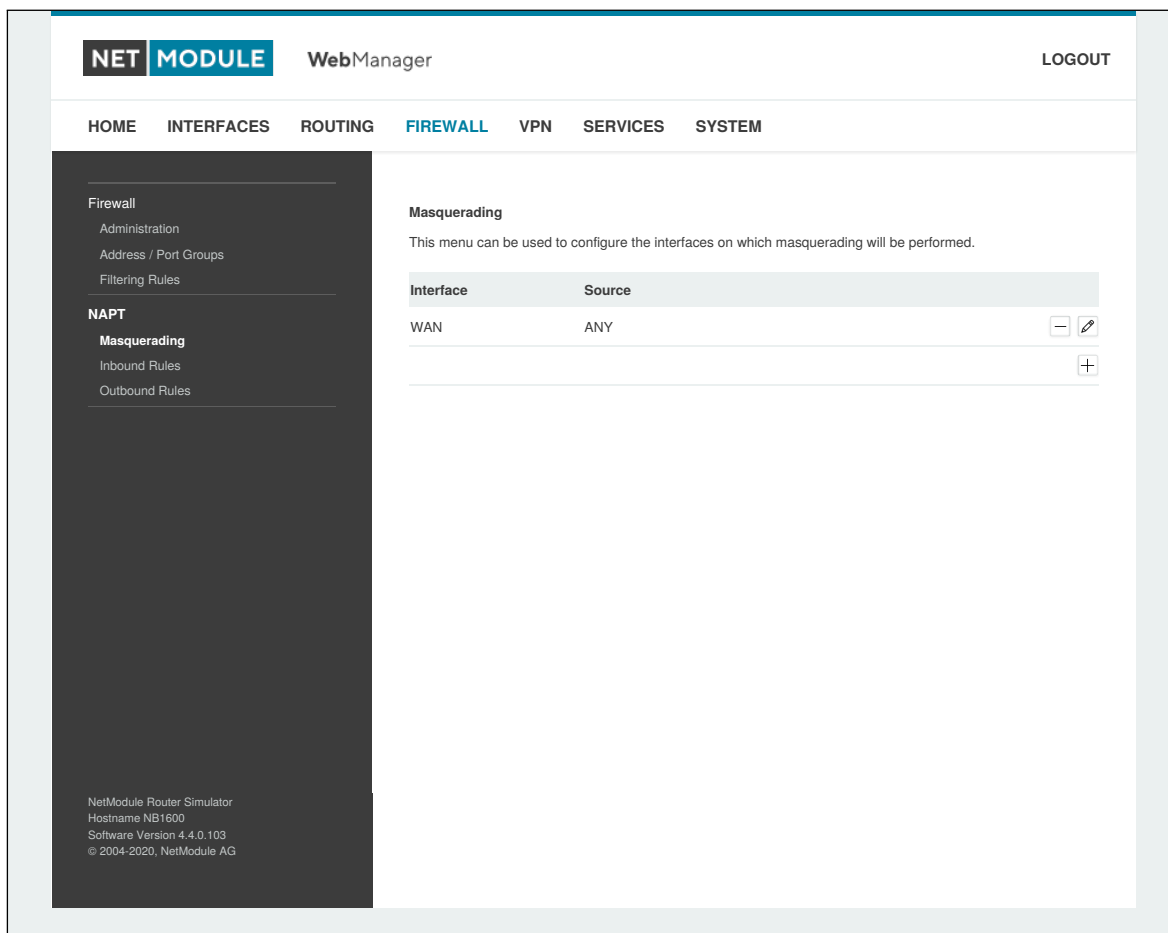
Abbildung 5.30.: Maskierung (Masquerading)
