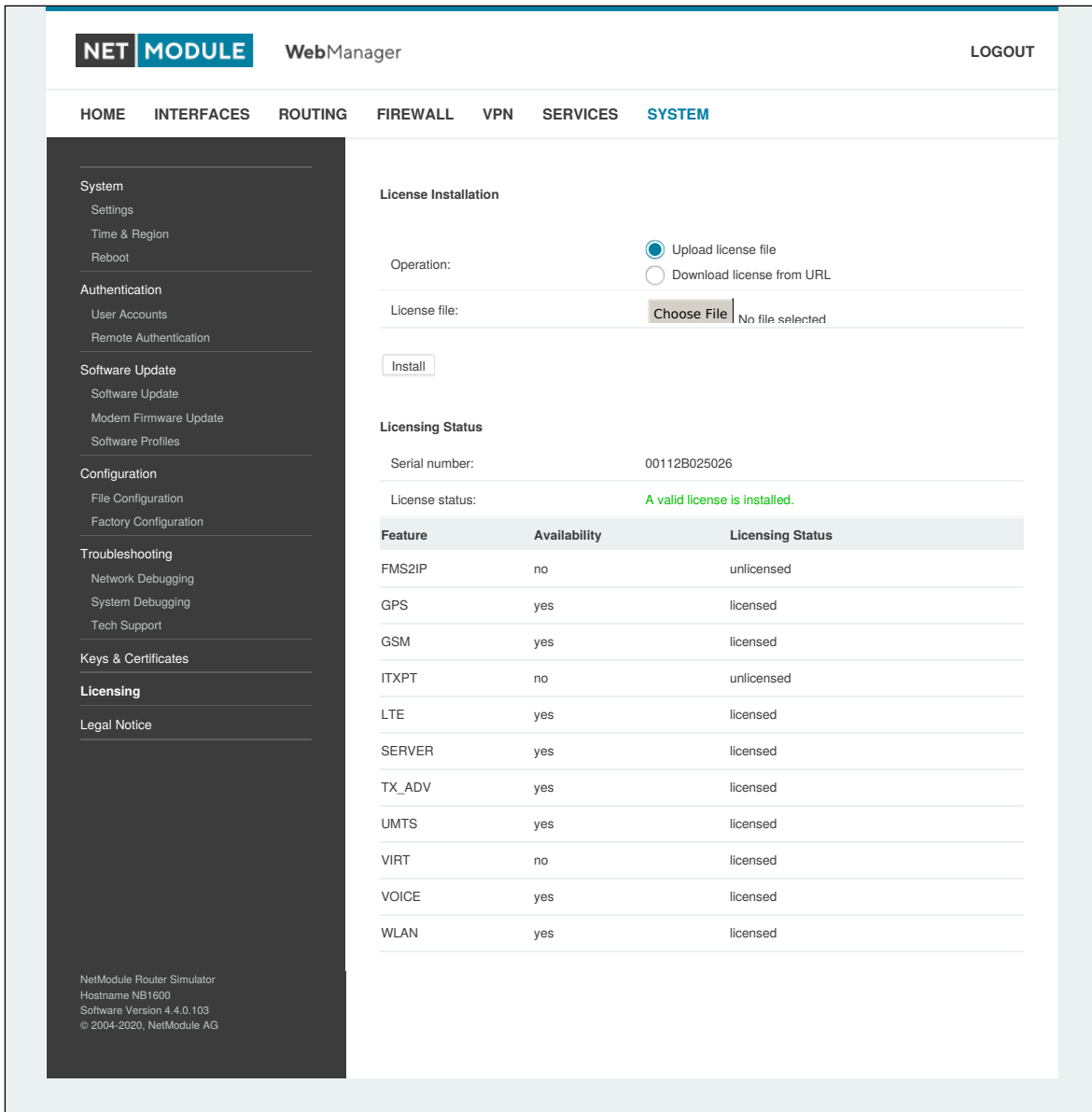
Abbildung 5.73.: Lizenzierung
