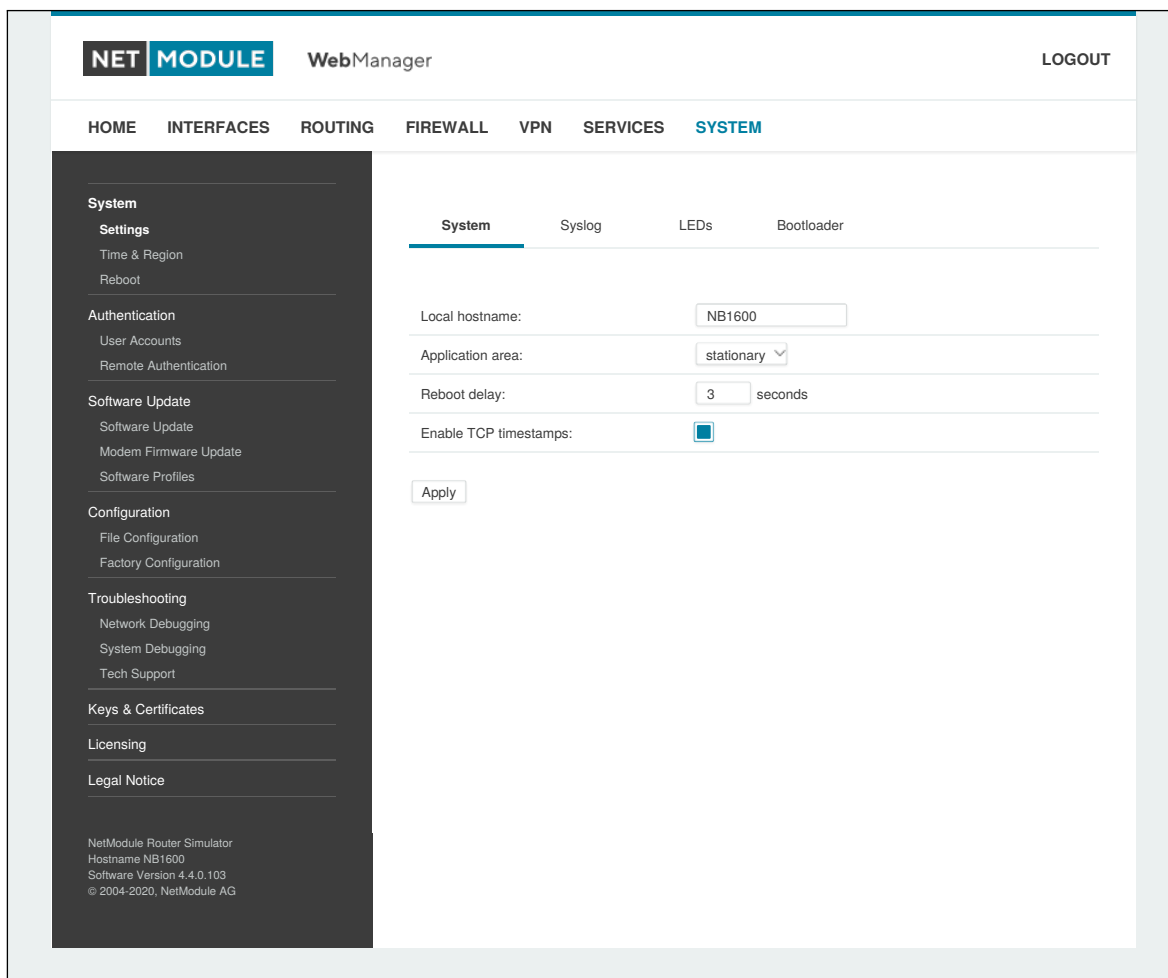
Abbildung 5.62.: System
