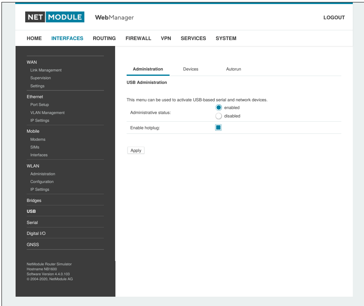
Abbildung 5.17.: USB-Verwaltung
