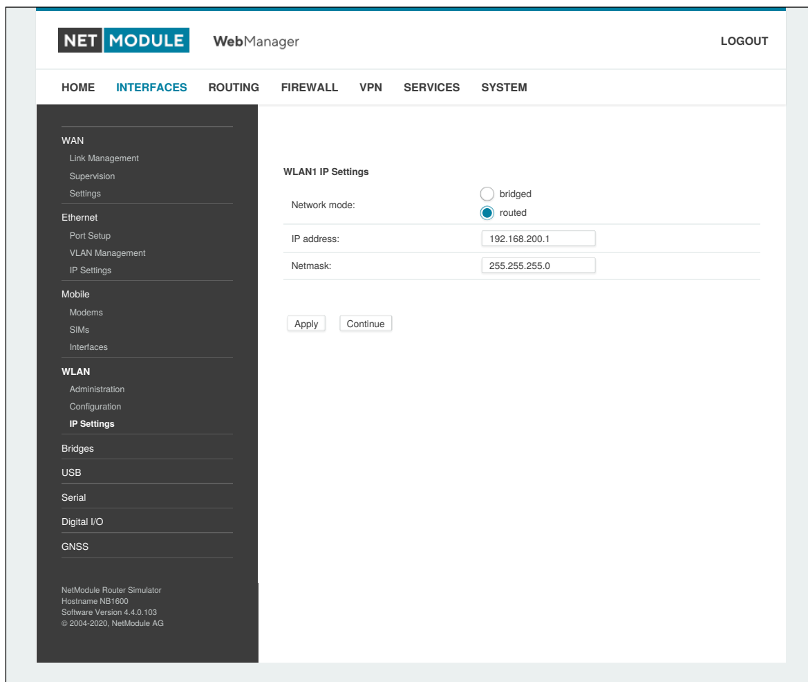
Abbildung 5.16.: WLAN-IP-Konfiguration
