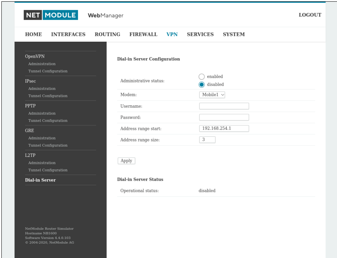
Abbildung 5.38.: Einwahlserver-Einstellungen
