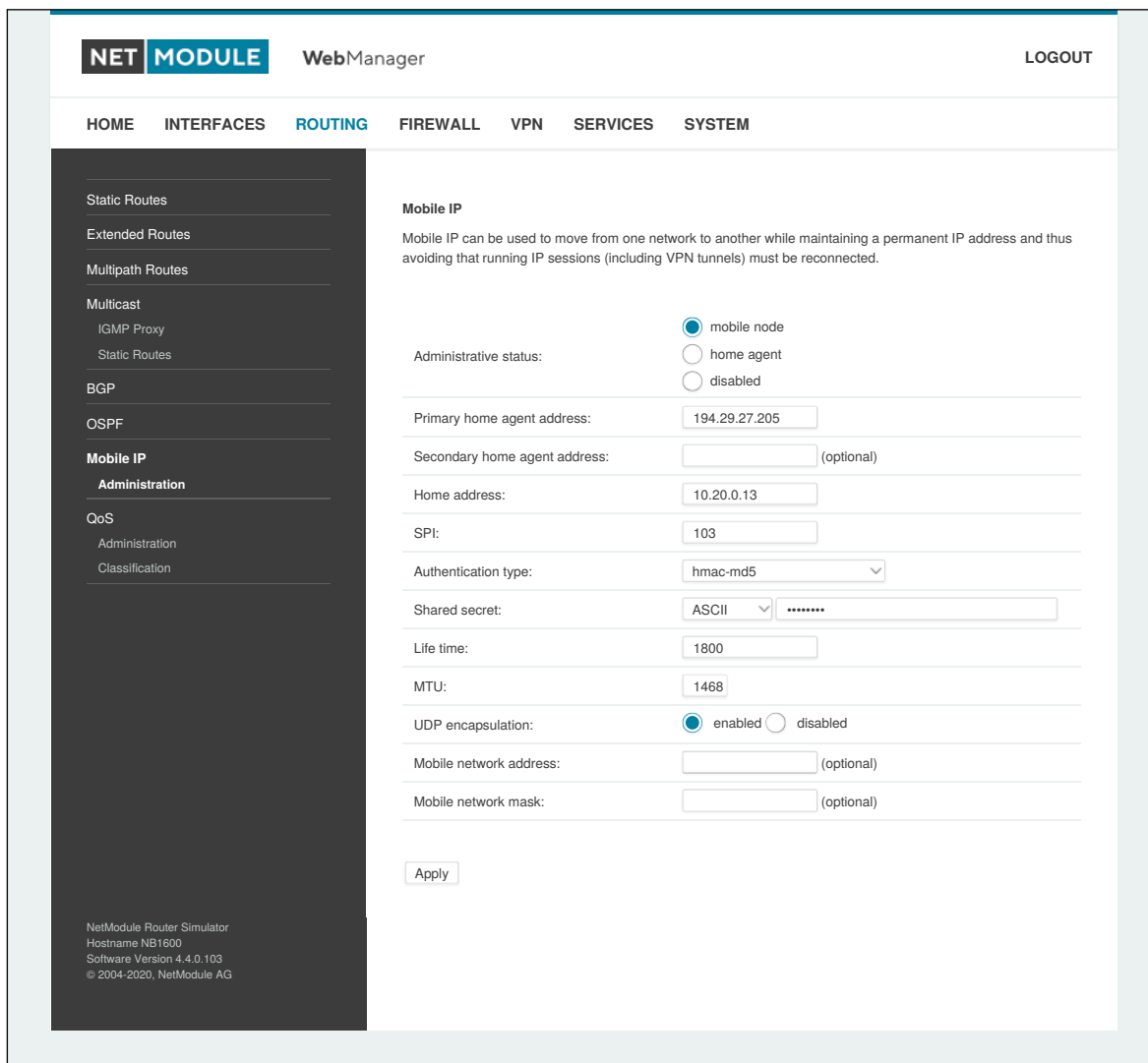
Abbildung 5.24.: Mobile IP
