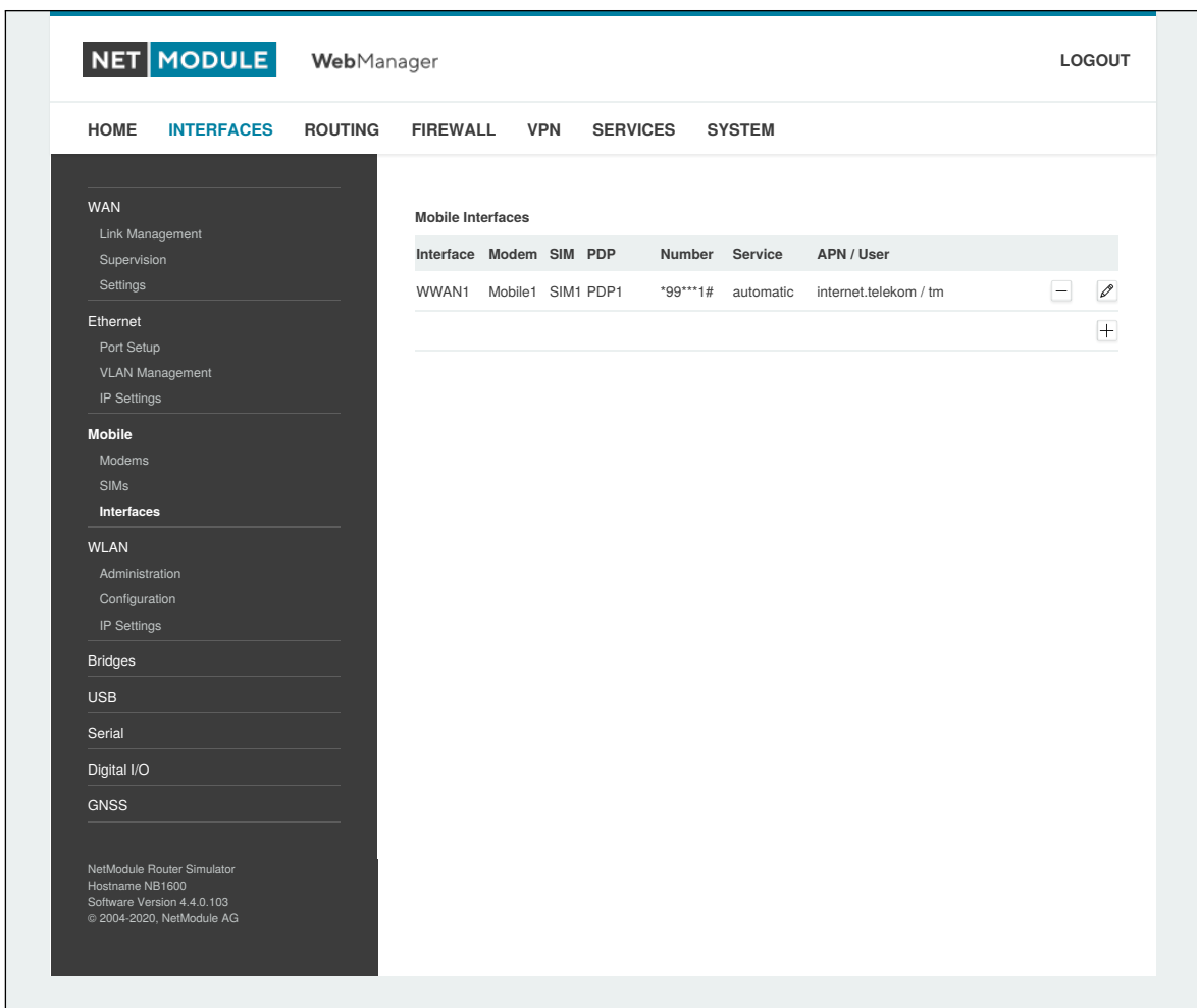
Abbildung 5.13.: WWAN-Schnittstellen
