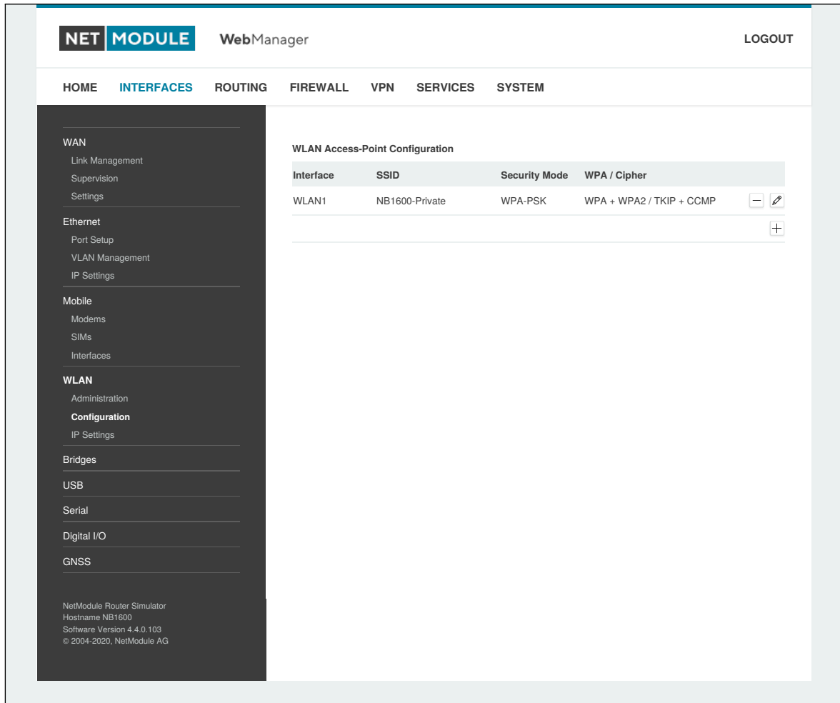
Abbildung 5.15.: WLAN-Konfiguration
