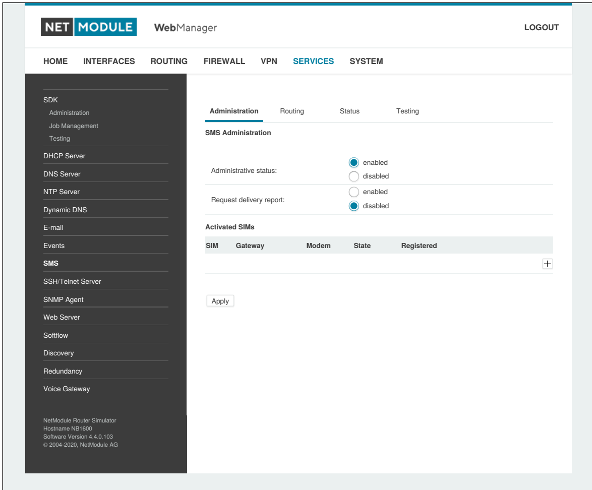
Abbildung 5.46.: SMS-Konfiguration
