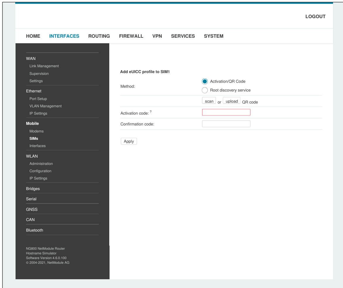
Abbildung 5.12.: eUICC-Profil hinzufügen
