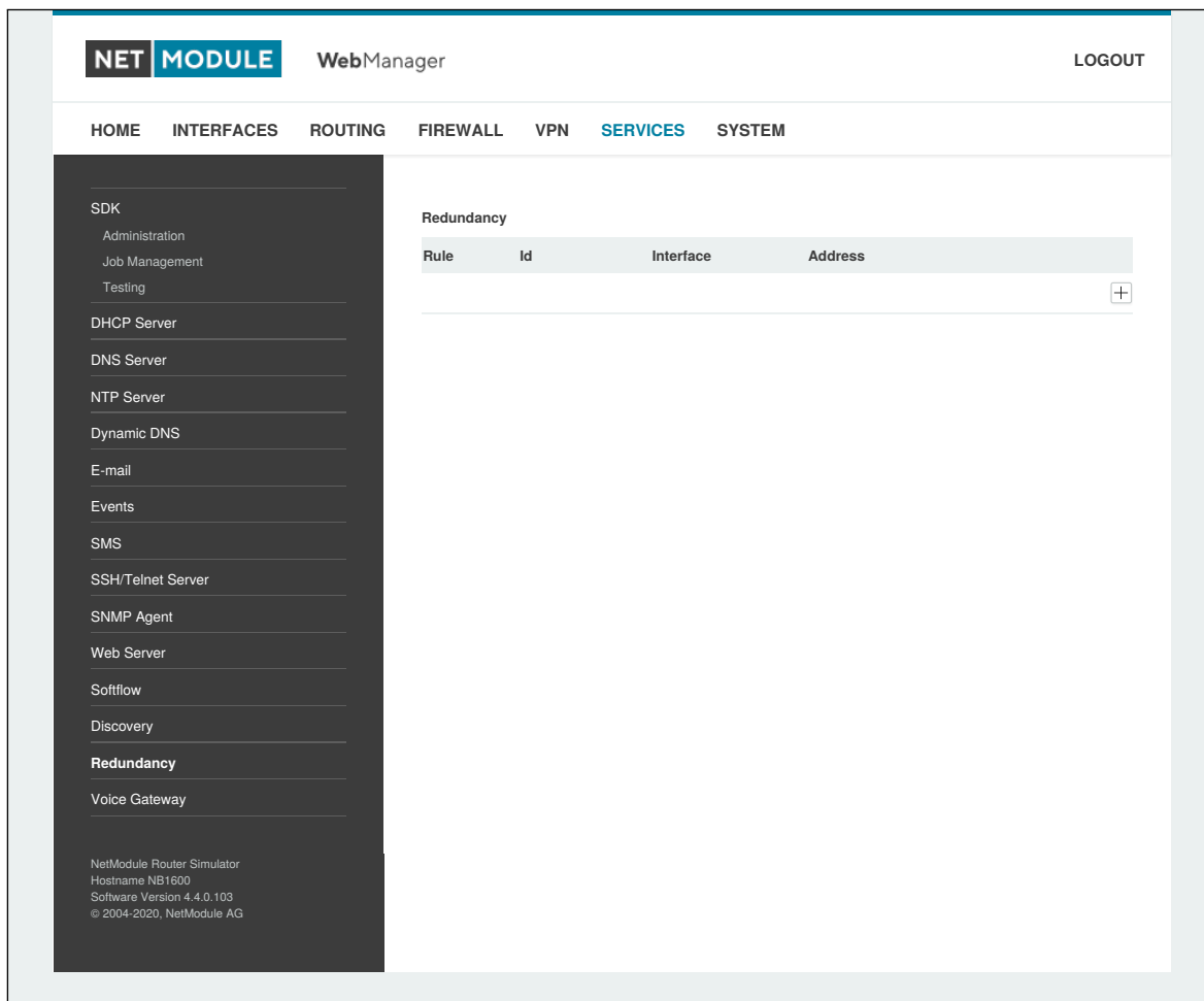
Abbildung 5.50.: VRRP-Konfiguration
