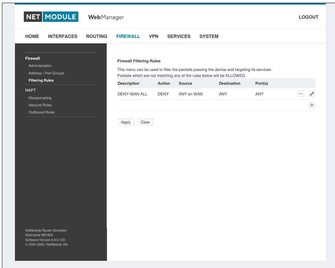
Abbildung 5.27.: Firewall-Regeln
