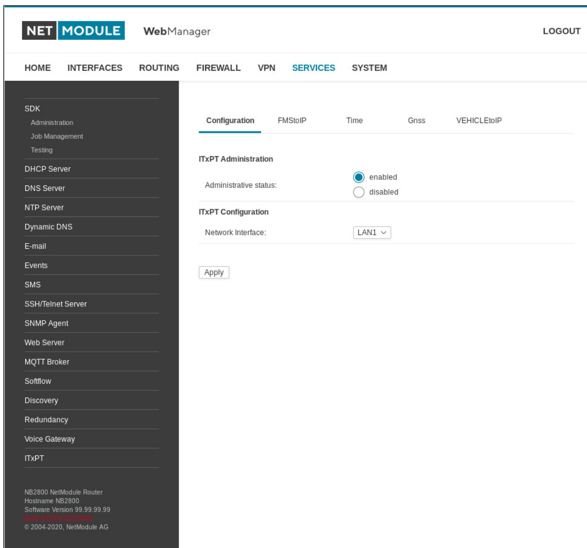
Abbildung 5.51.: ITxPT-Konfiguration
