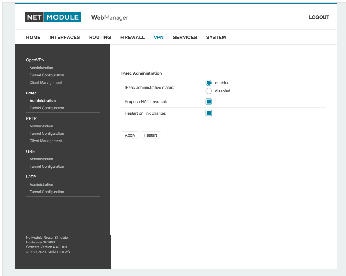
Abbildung 5.33.: IPsec-Verwaltung
