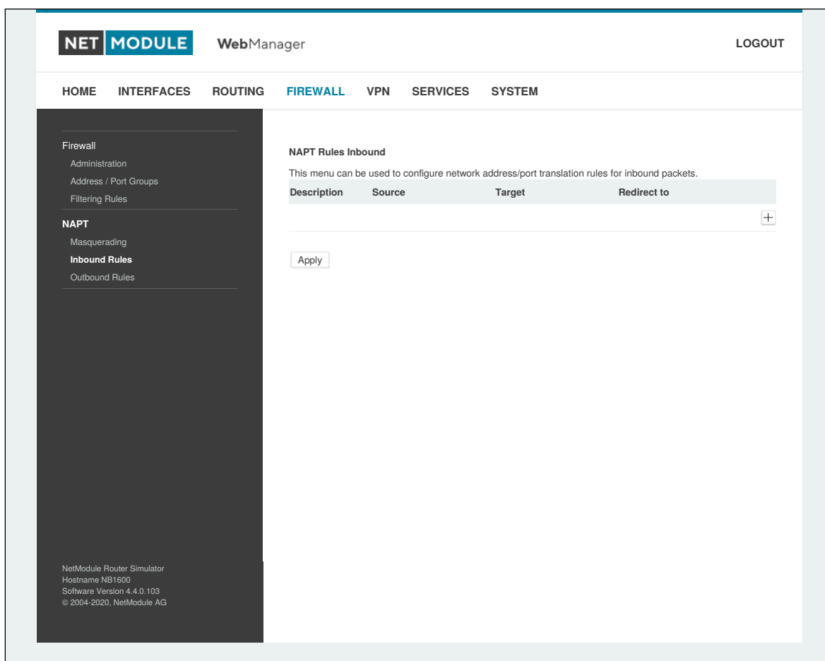
Abbildung 5.27.: NAPT-Regeln für eingehende Pakete
