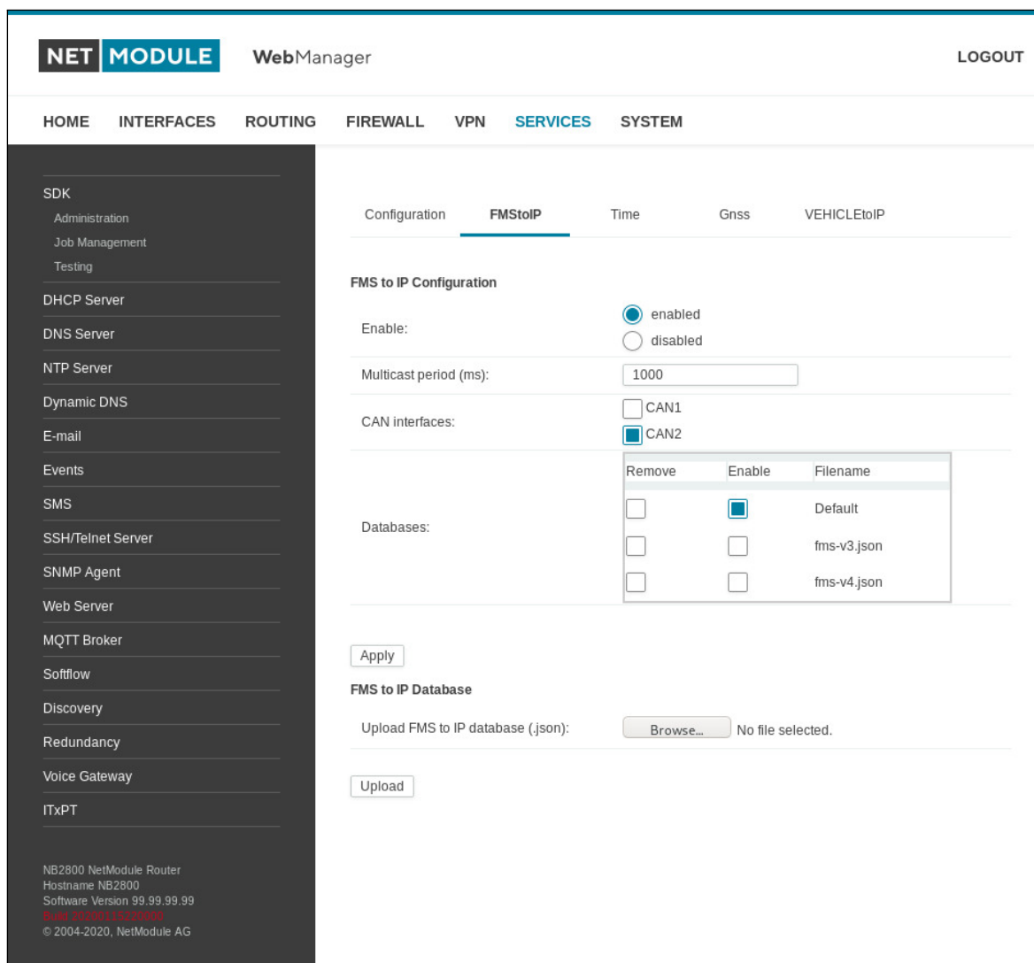
Abbildung 5.50.: ITxPT FMS-to-IP
