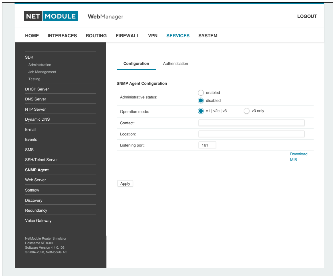
Abbildung 5.46.: SNMP-Agent
