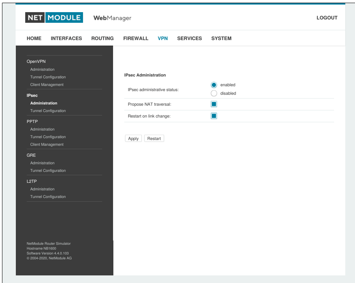
Abbildung 5.31.: IPSec-Verwaltung
