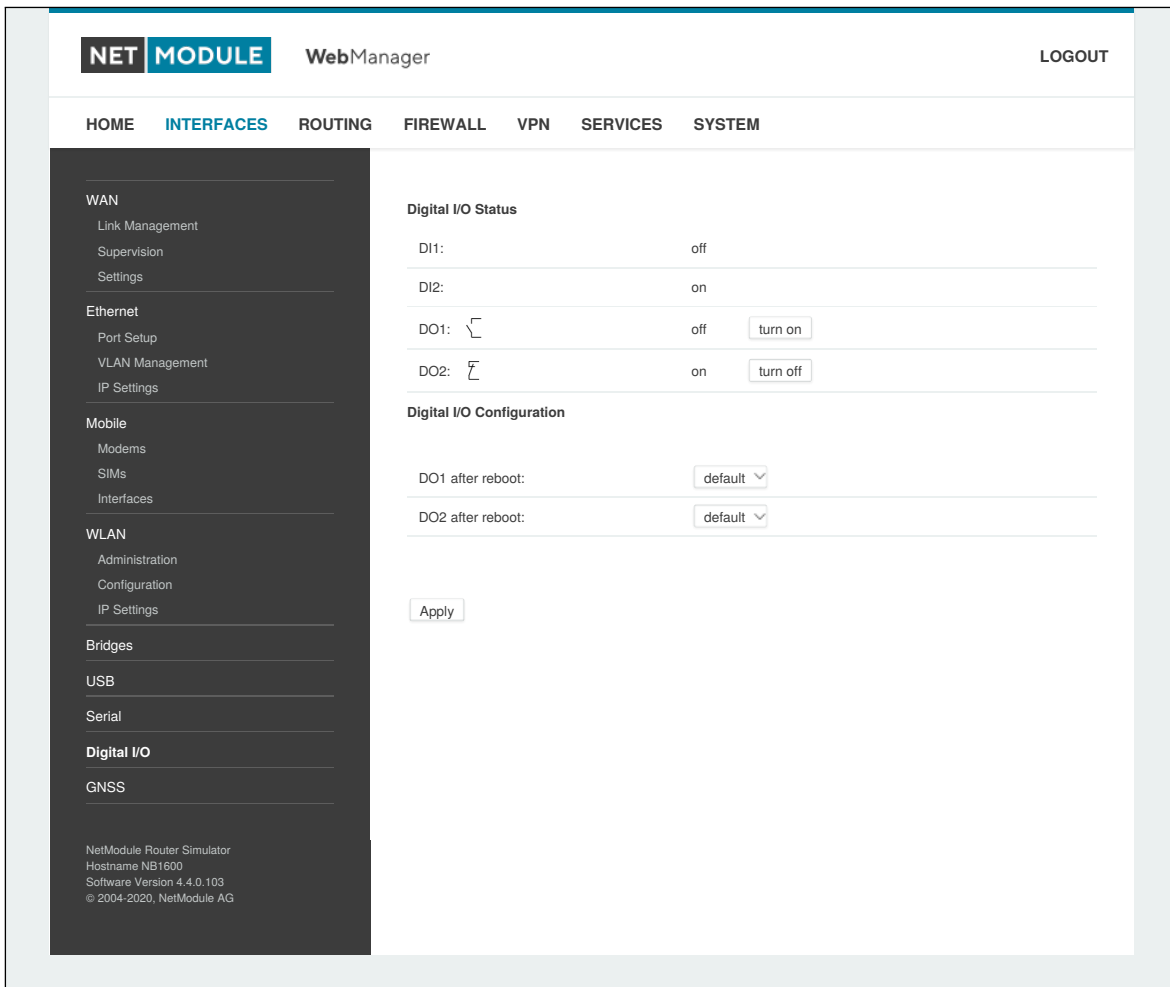
Abbildung 5.19.: Digitale Ein-/Ausgänge
