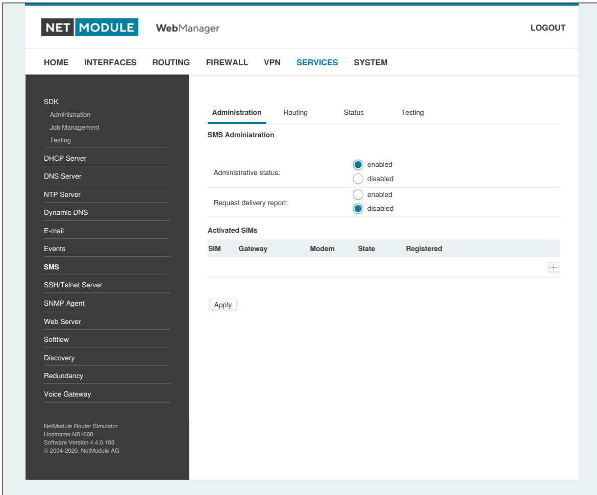
Abbildung 5.44.: SMS-Konfiguration
