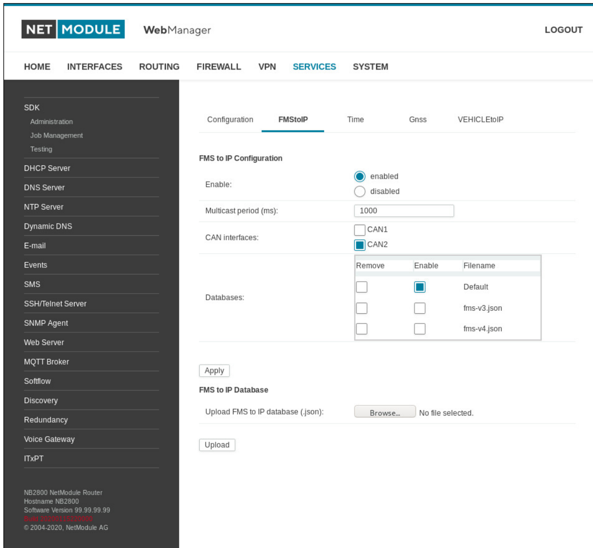
Abbildung 5.50.: ITxPT FMS-to-IP
