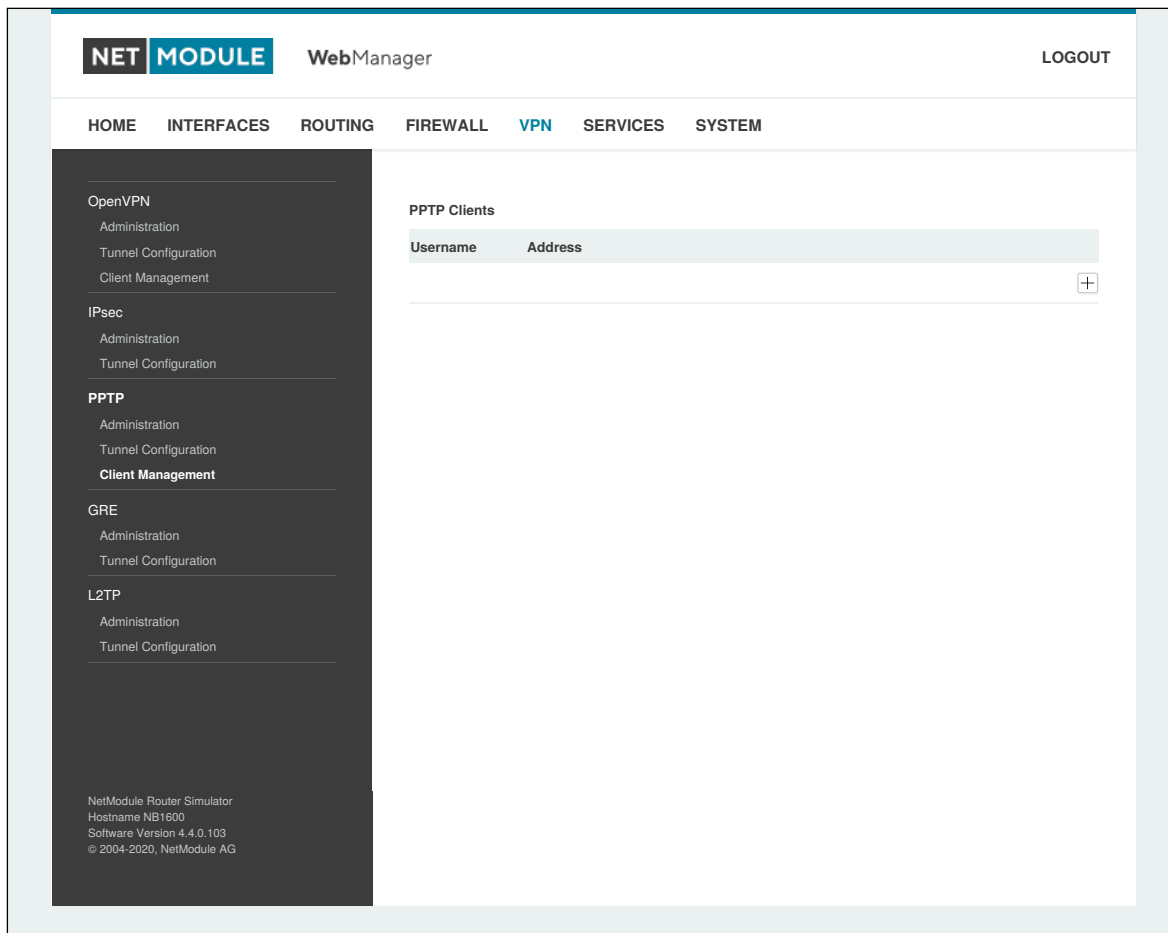
Abbildung 5.34.: PPTP-Client-Verwaltung
