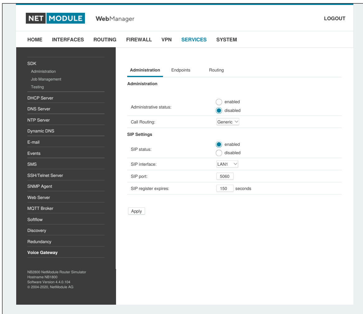
Abbildung 5.49.: Verwaltung des Voice-Gateways
