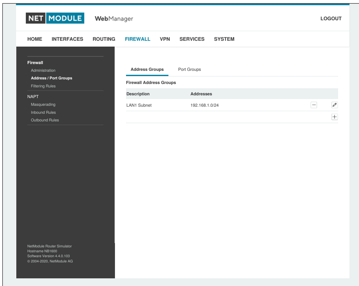
Abbildung 5.24.: Firewall-Gruppen
