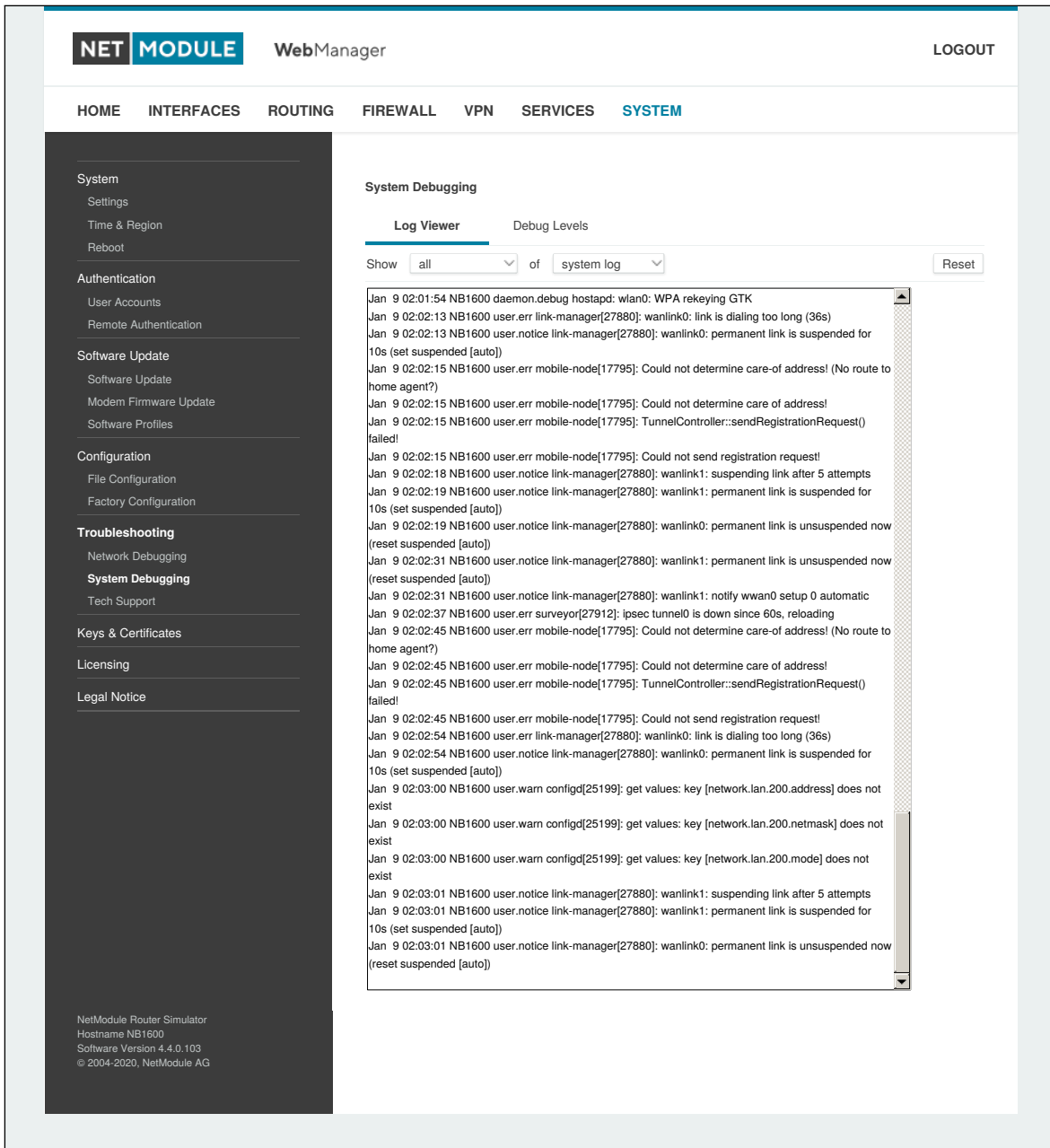
Abbildung 5.57.: Log-Viewer
