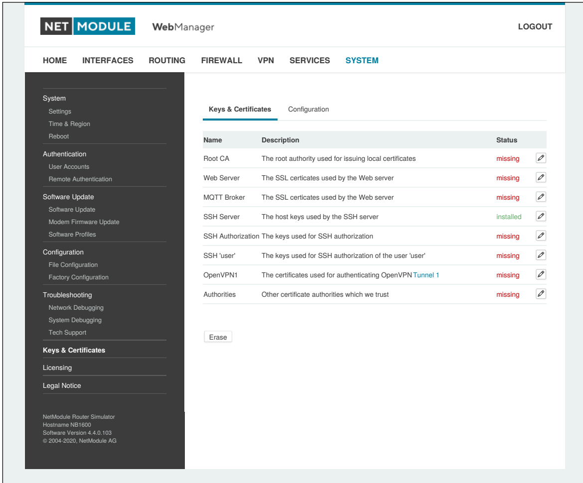
Abbildung 5.59.: Schlüssel und Zertifikate
