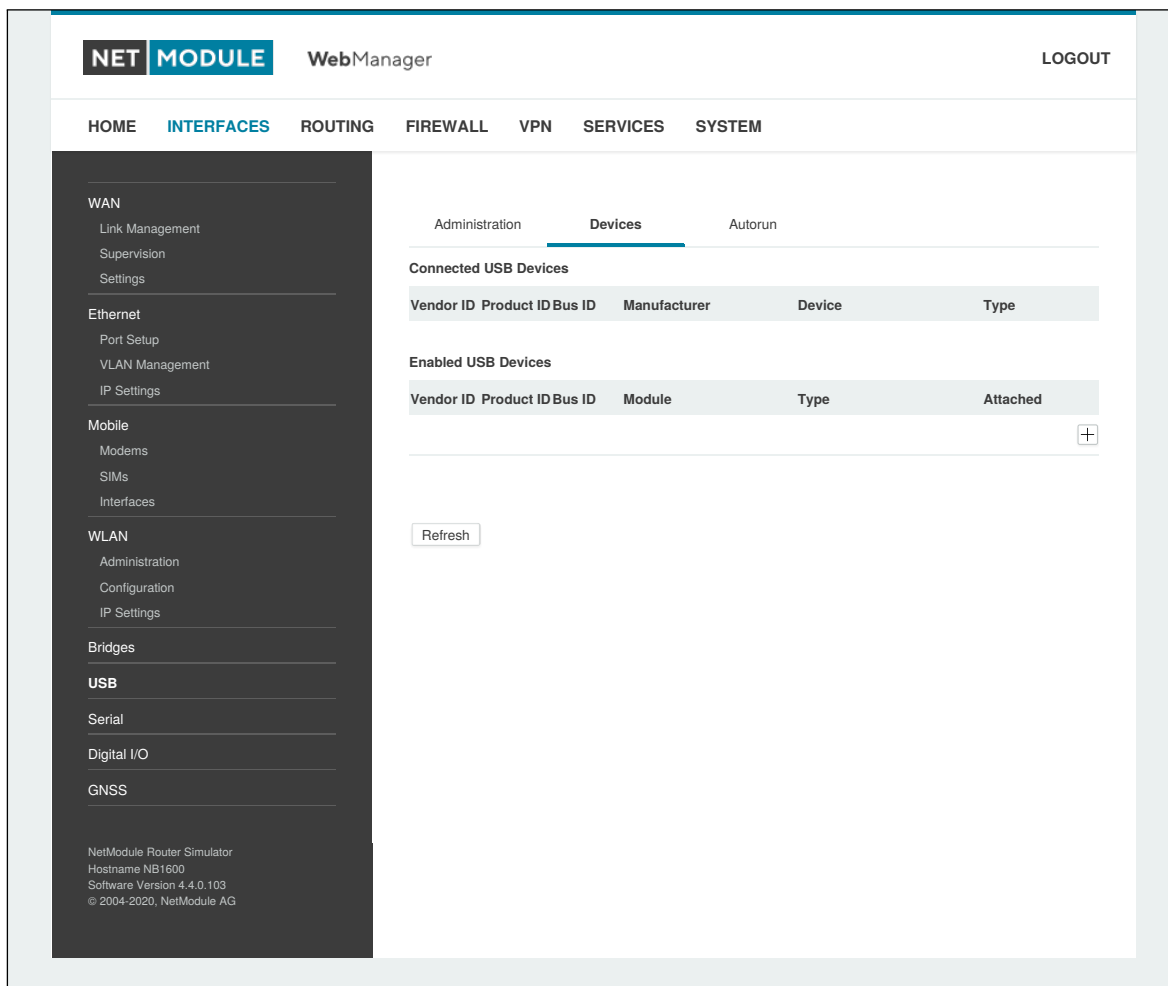
Abbildung 5.16.: USB-Geräteverwaltung
