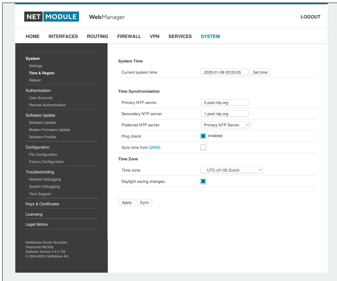
Abbildung 5.51.: Regionseinstellungen
