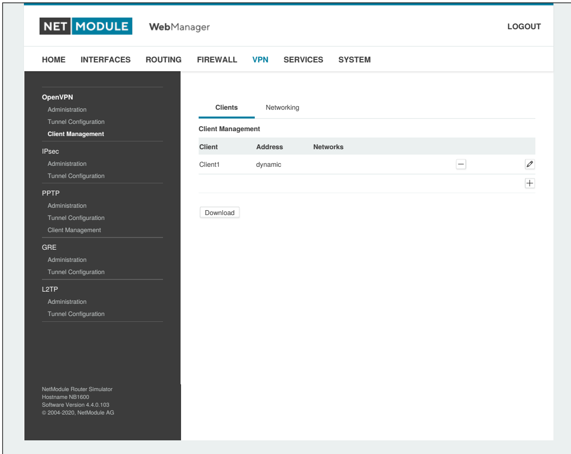
Abbildung 5.30.: OpenVPN-Client-Verwaltung
