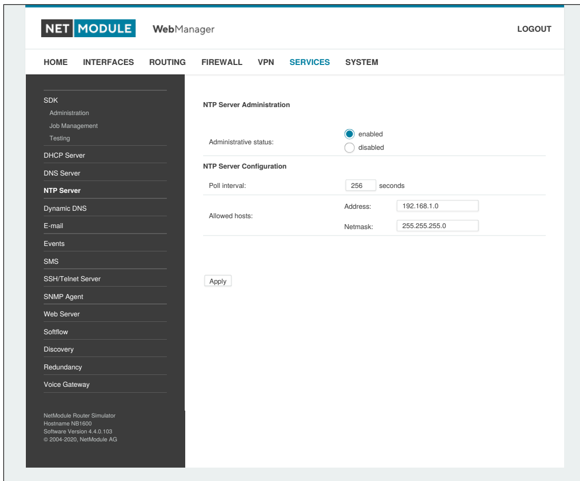
Abbildung 5.41.: NTP-Server
