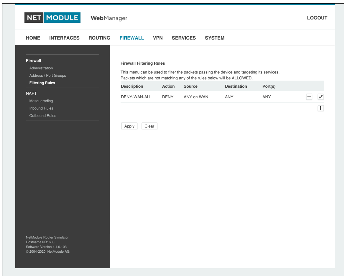
Abbildung 5.25.: Firewall-Regeln
