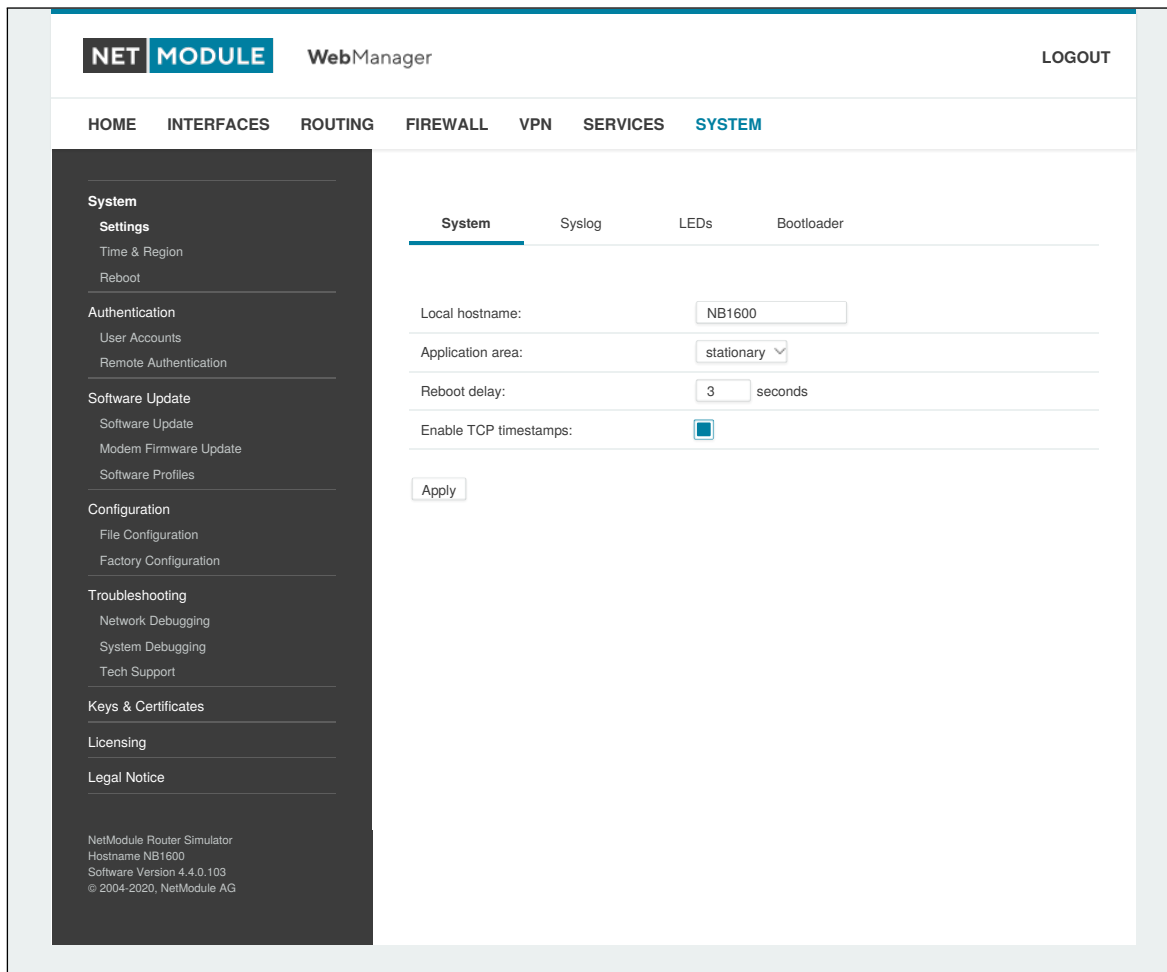
Abbildung 5.54.: System
