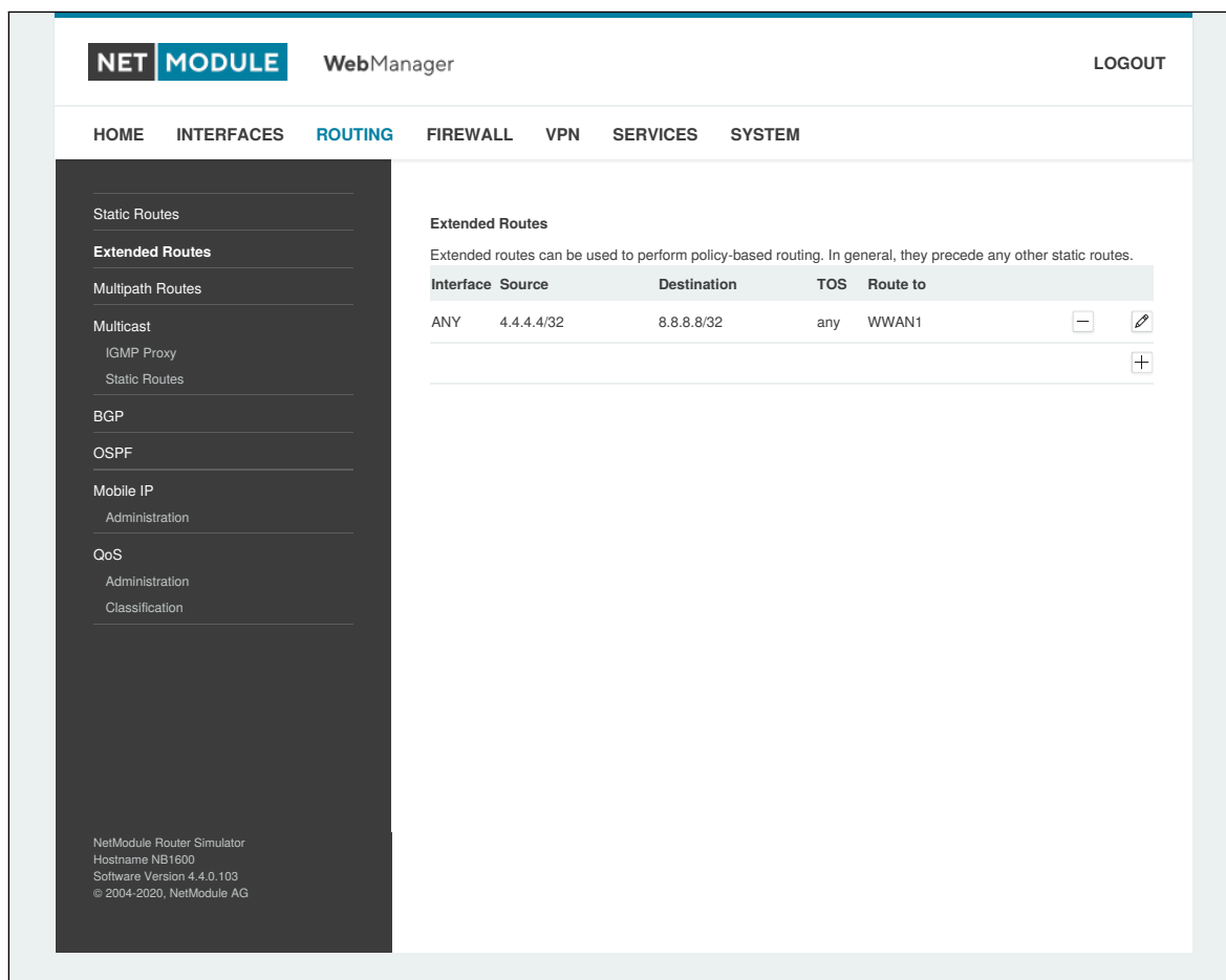
Abbildung 5.20.: Erweitertes Routing
