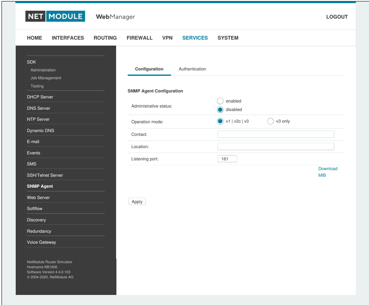
Abbildung 5.45.: SNMP-Agent
