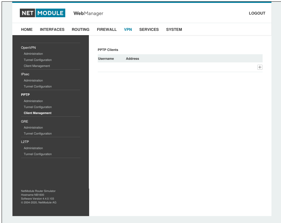
Abbildung 5.34.: PPTP-Client-Verwaltung
