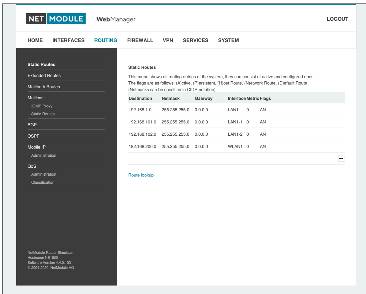
Abbildung 5.20.: Statisches Routing
