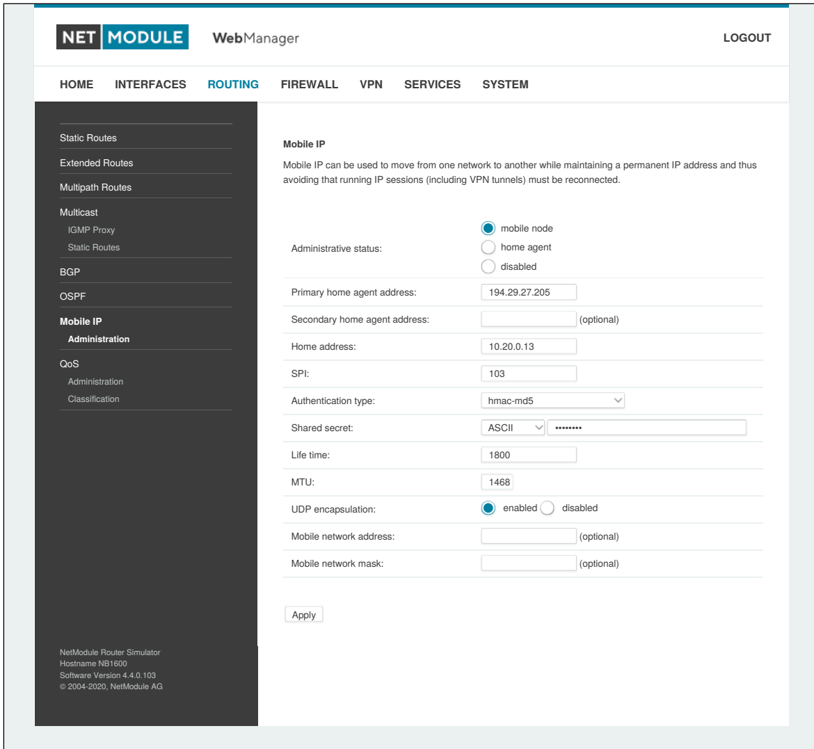
Abbildung 5.23.: Mobile IP
