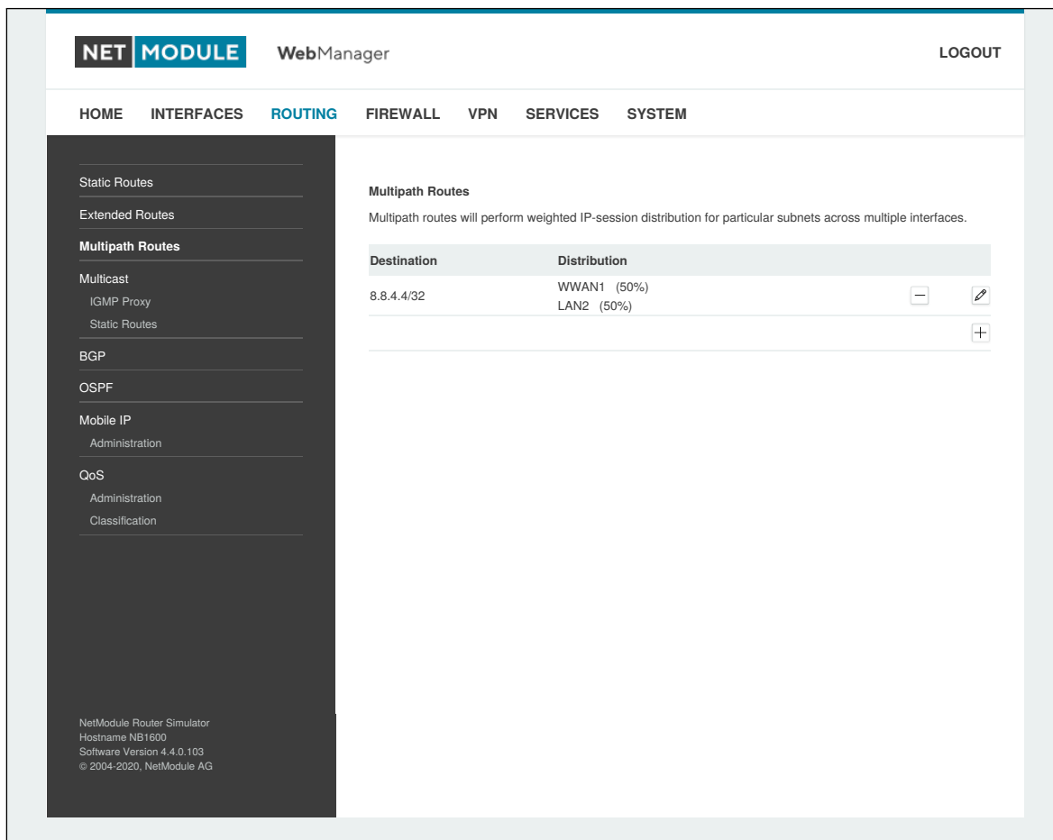
Abbildung 5.22.: Multipath-Routing
