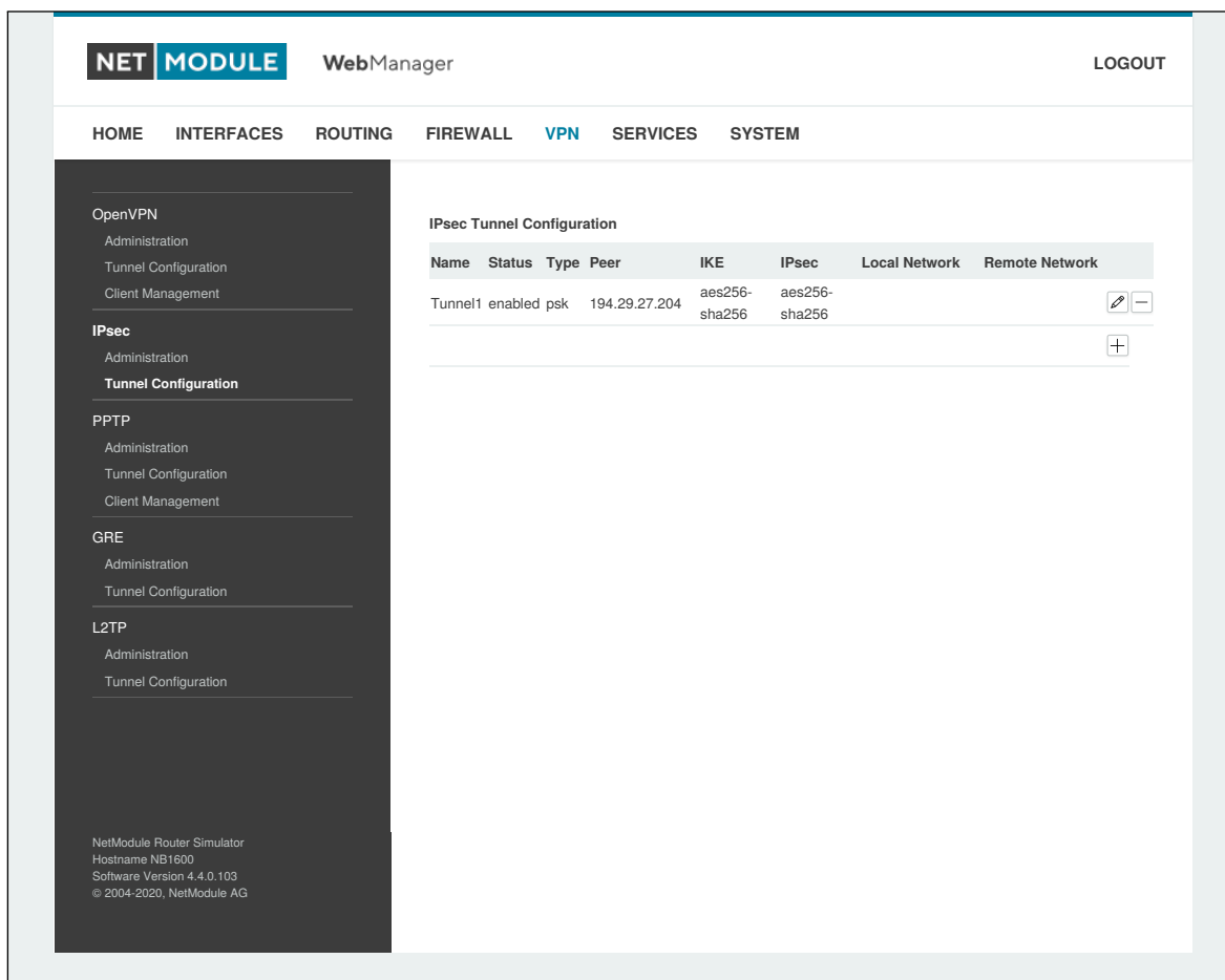
Abbildung 5.32.: IPsec-Konfiguration
