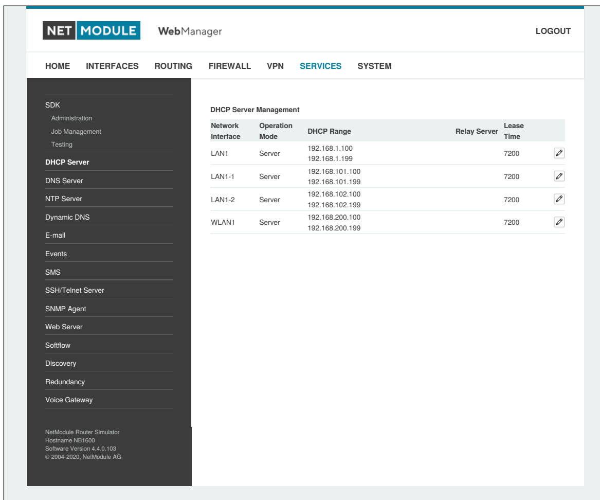
Abbildung 5.39.: DHCP-Server
