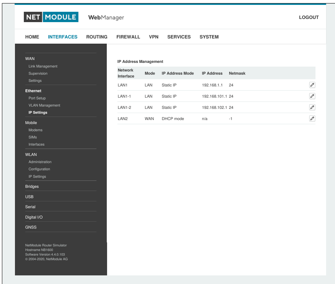
Abbildung 5.9.: LAN-IP-Konfiguration
