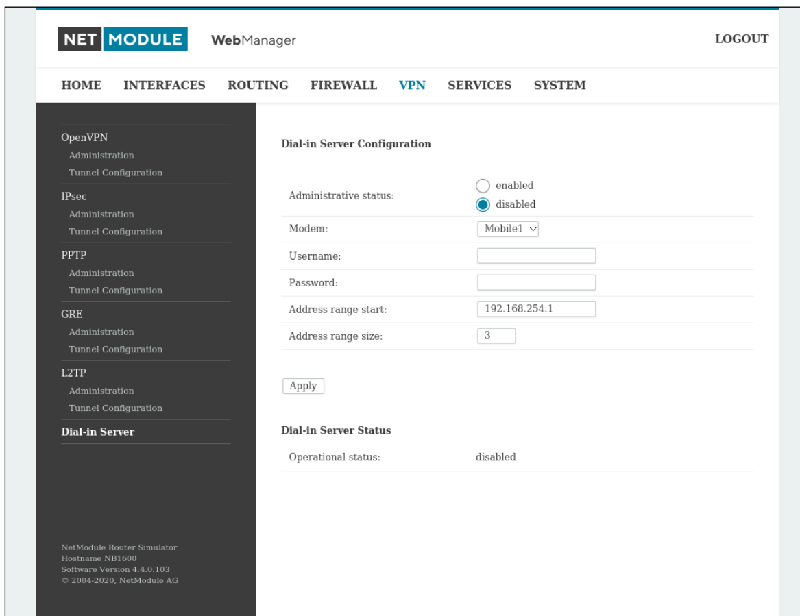
Abbildung 6.40.: Einwahlserver-Einstellungen
