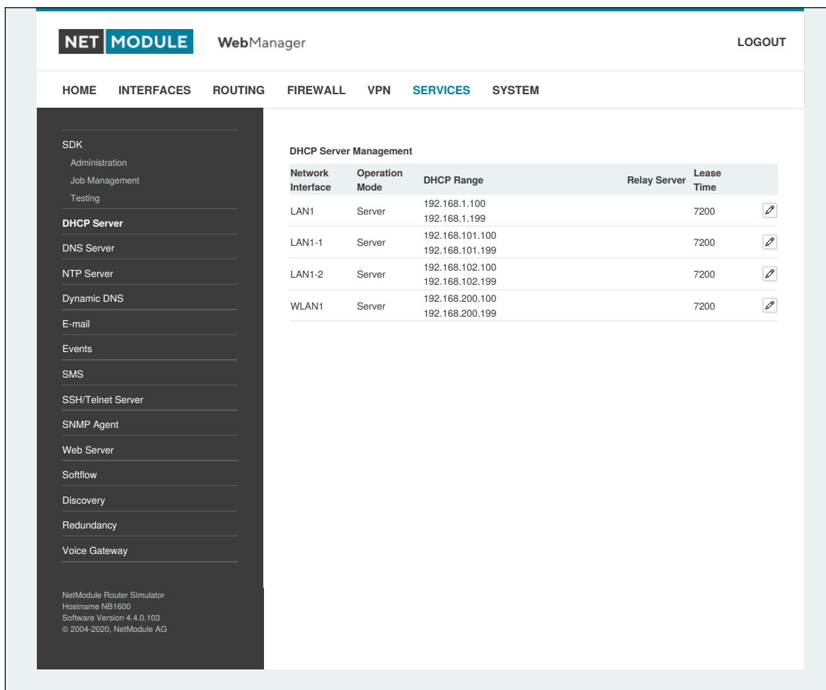
Abbildung 6.43.: DHCP-Server
