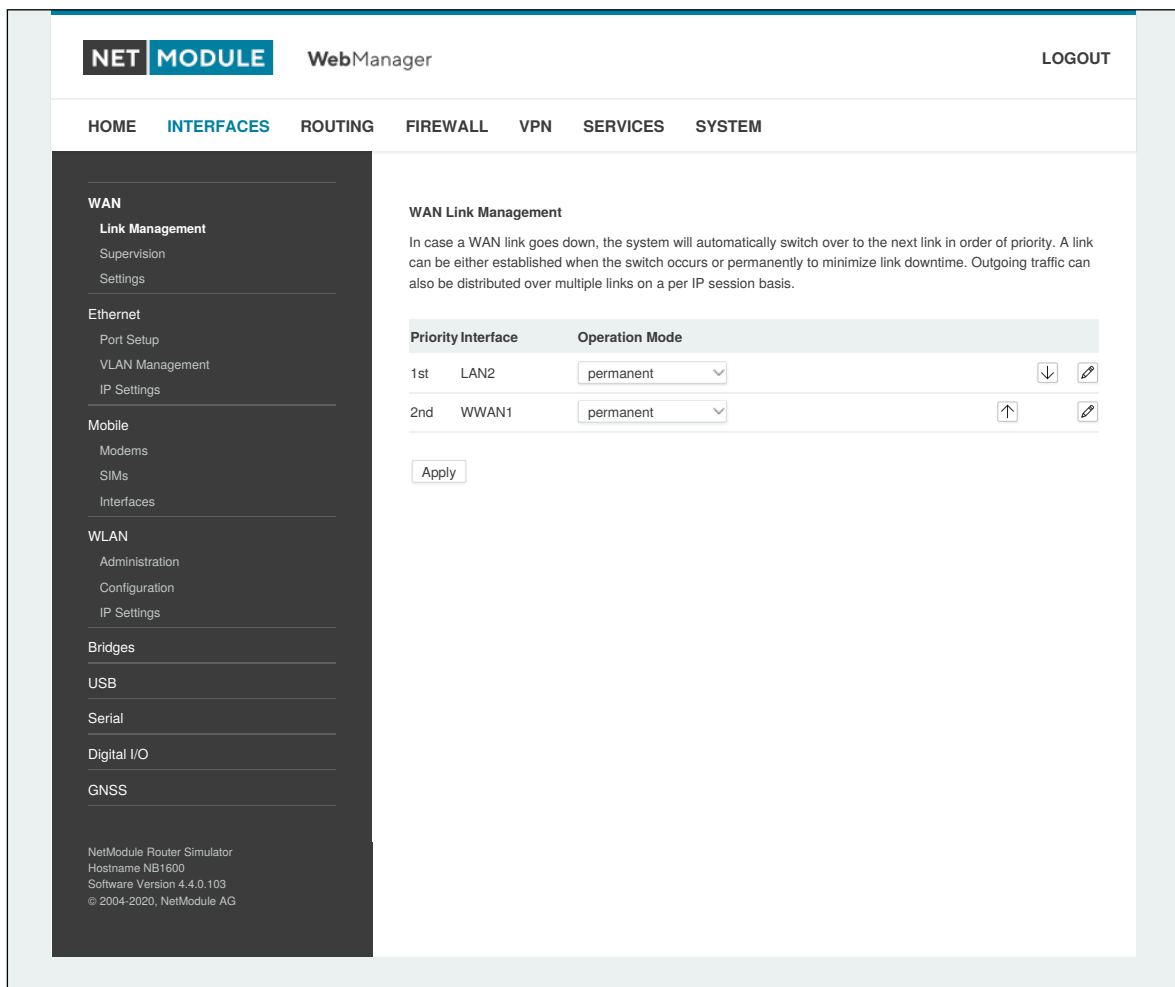
Abbildung 6.3.: WAN-Verbindungen
