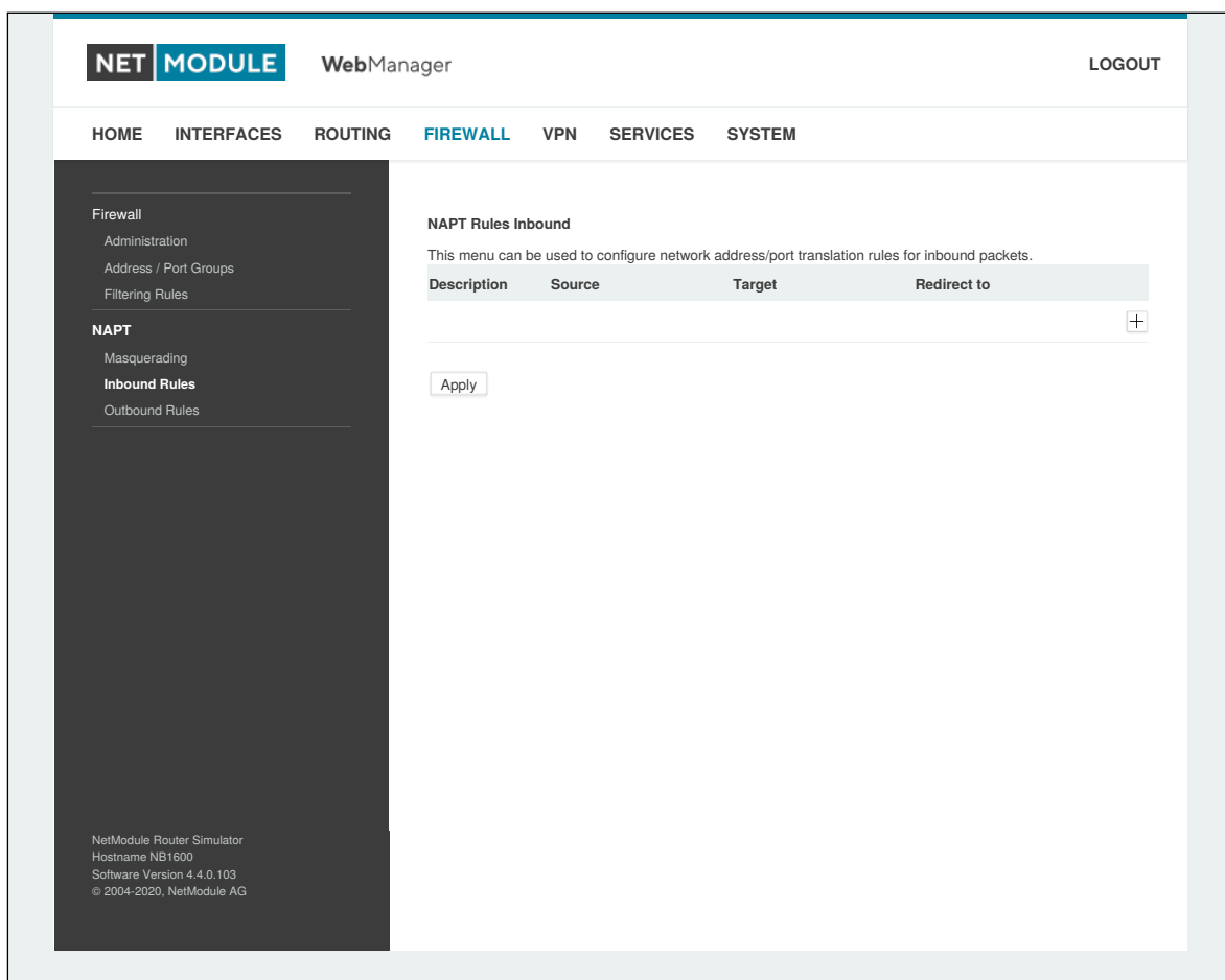
Abbildung 6.29.: NAPT-Regeln für eingehende Pakete
