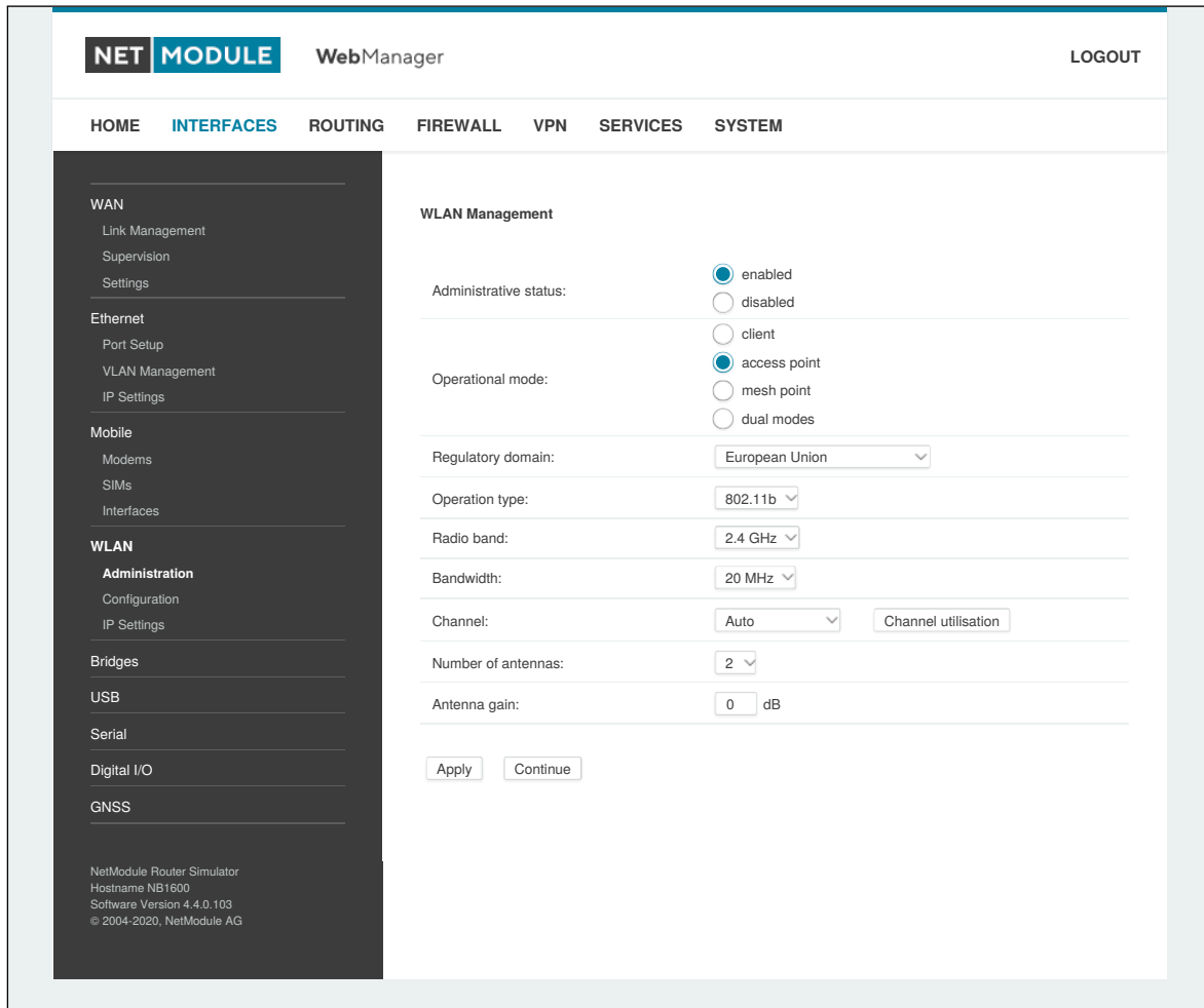
Abbildung 6.61.: WLAN administration
