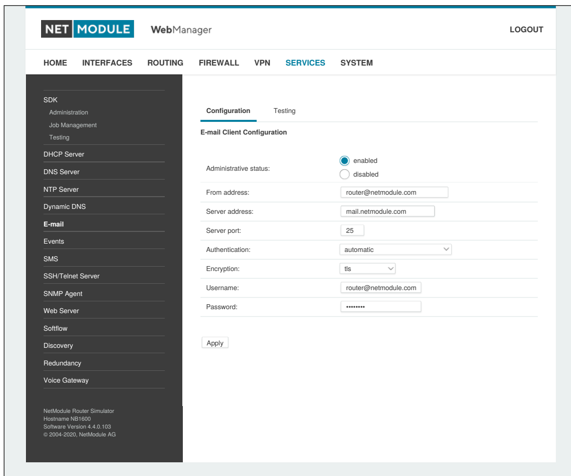
Abbildung 6.47.: E-Mail-Einstellungen
