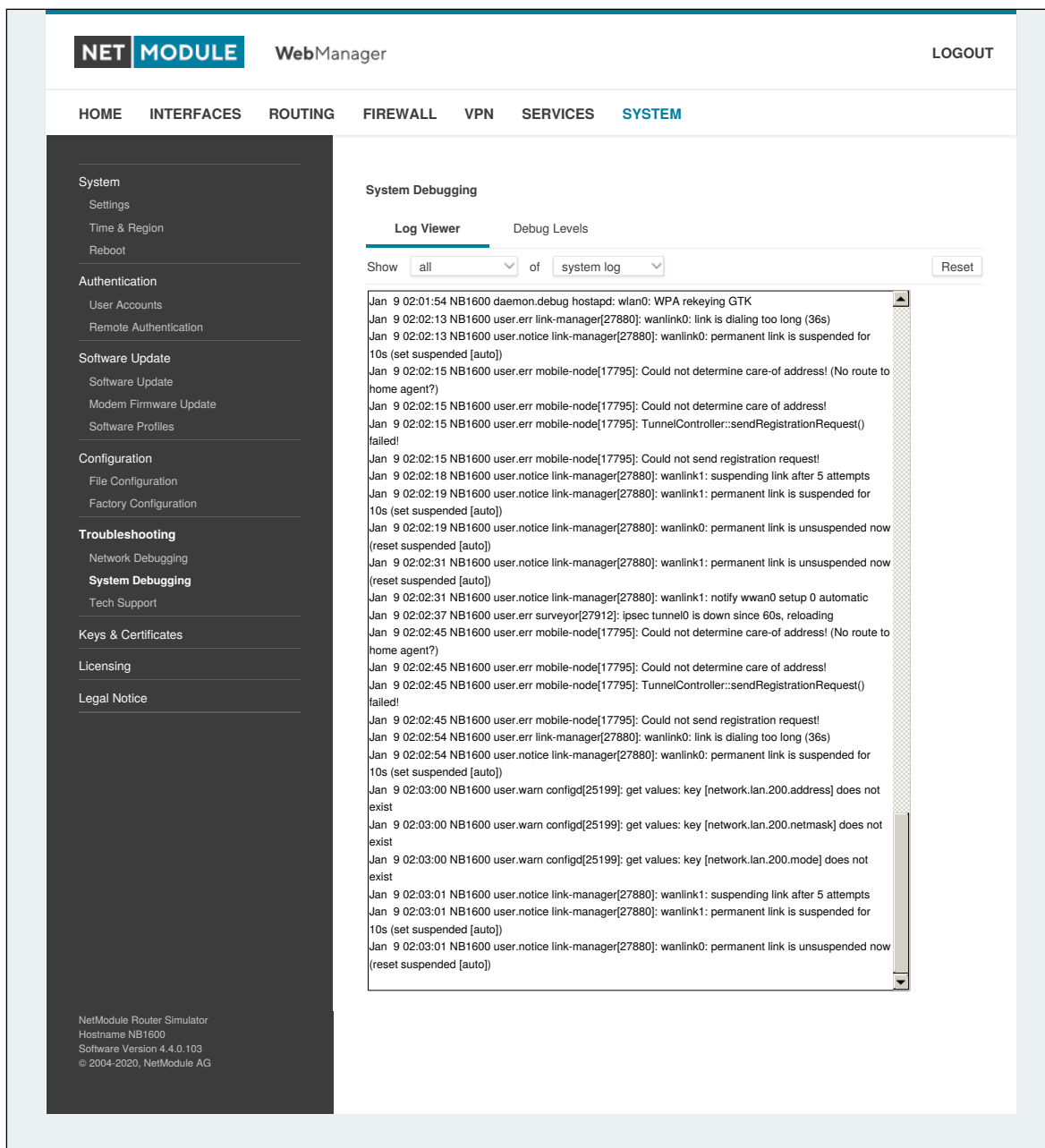
Abbildung 5.70.: Log-Viewer
