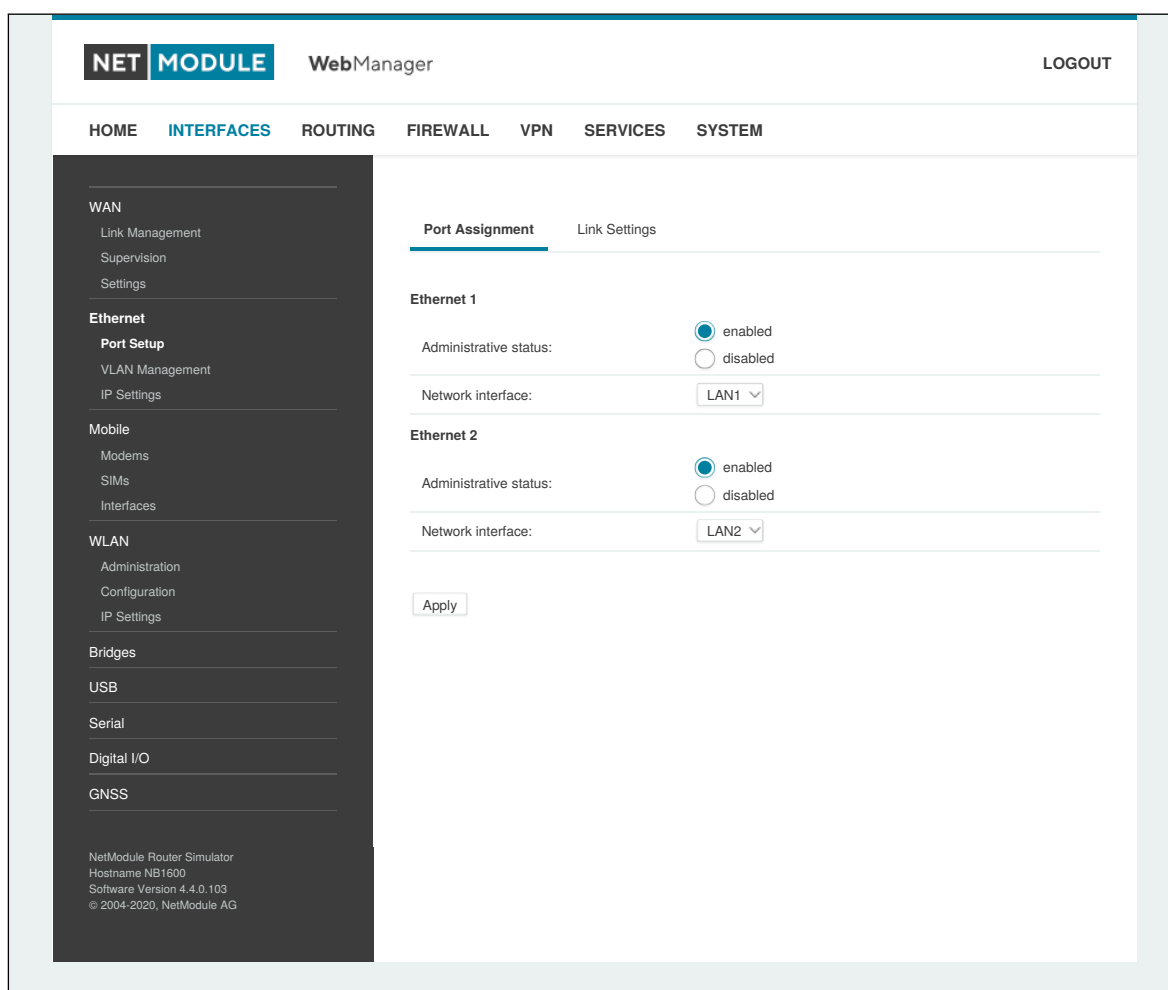
Abbildung 5.7.: Ethernet-Anschlüsse
