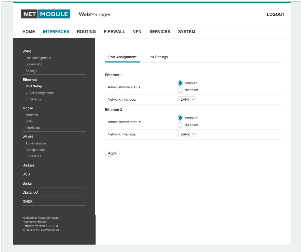
Abbildung 5.6.: Ethernet-Anschlüsse
