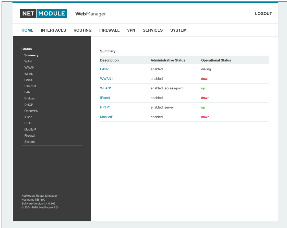
Abbildung 5.2.: Startbildschirm
