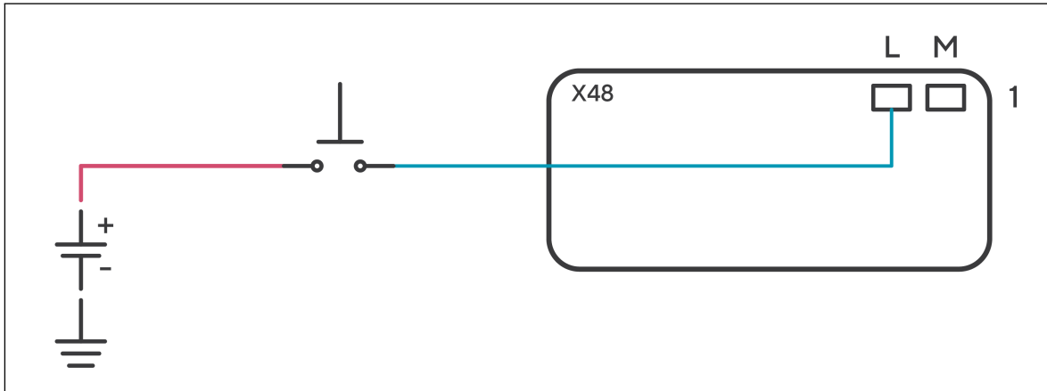
Abbildung 3.1.: Reset-Eingang (serielle Schnittstelle nicht verwendet)
