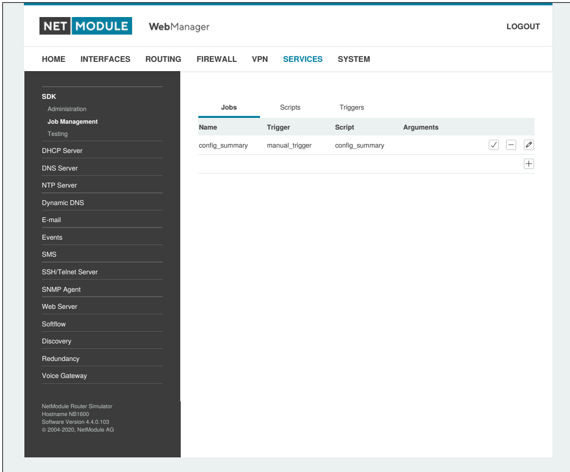
Abbildung 5.42.: SDK-Jobs
