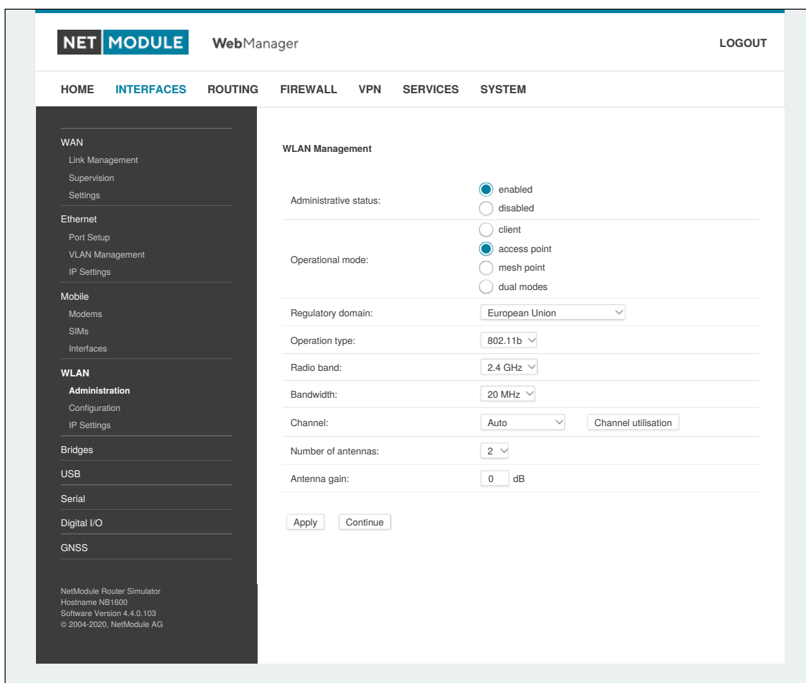
Abbildung 5.16.: WLAN-Verwaltung
