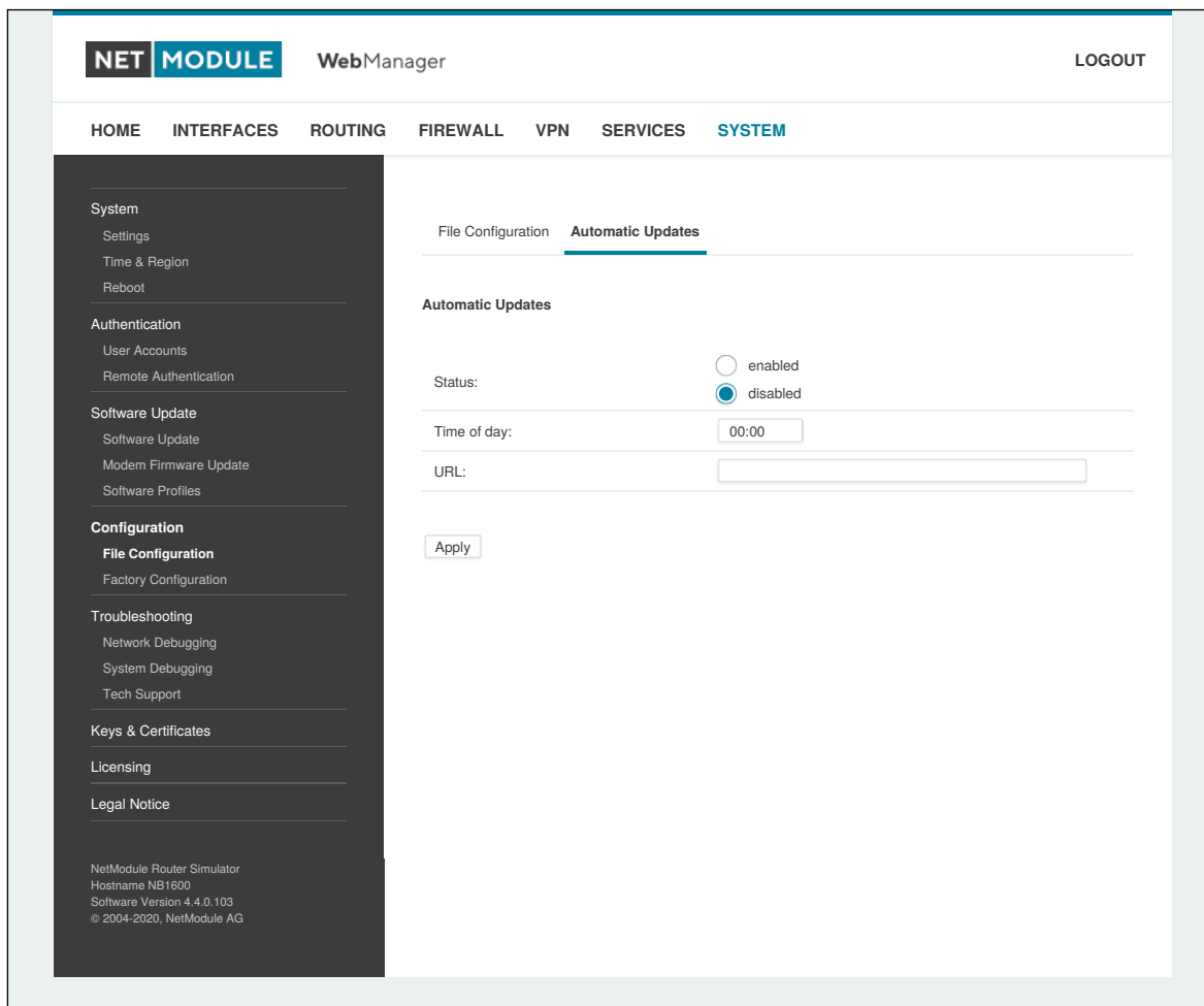
Abbildung 5.63.: Automatische Konfiguration per Datei
