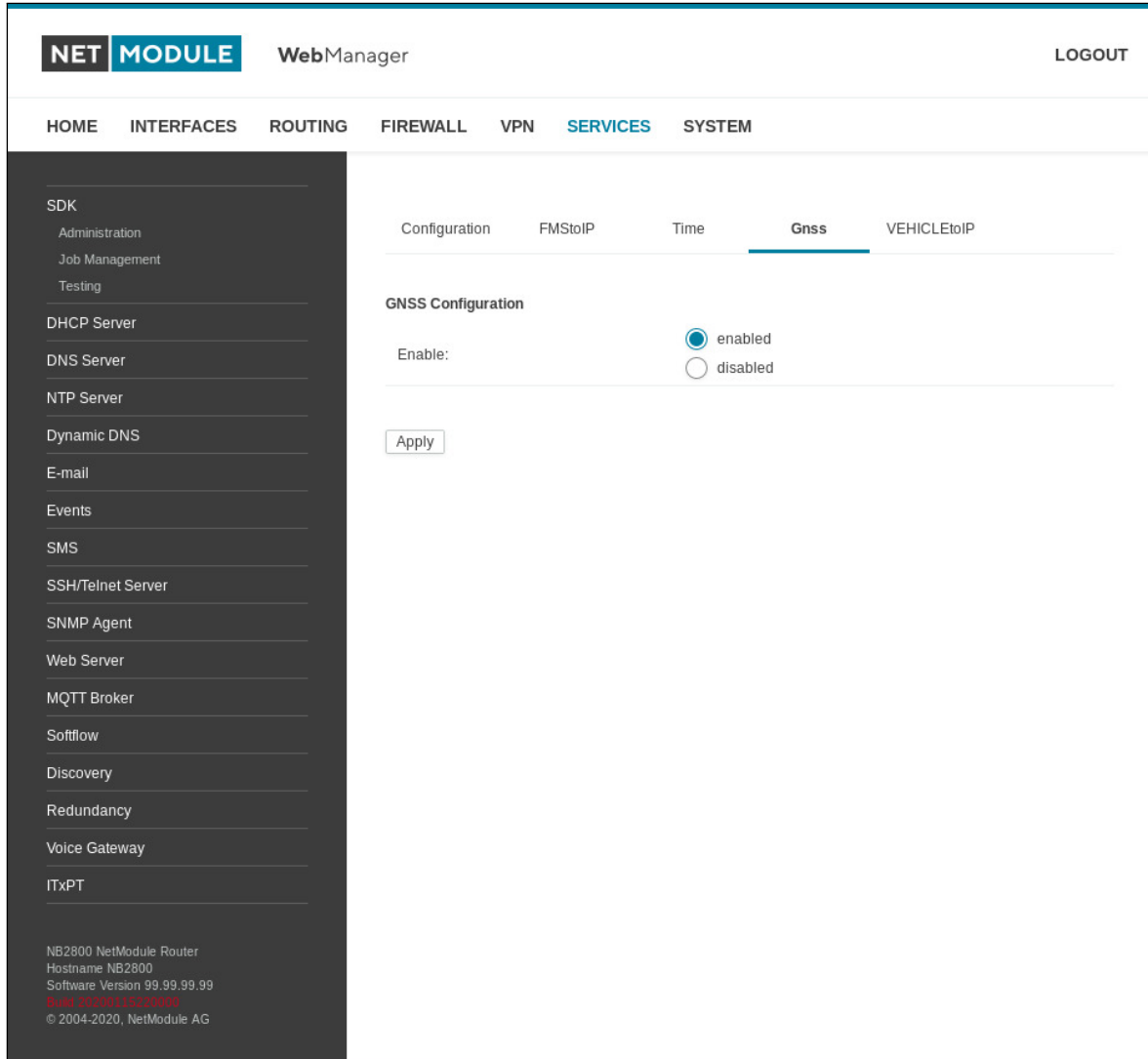
Abbildung 5.55.: ITxPT GNSS
