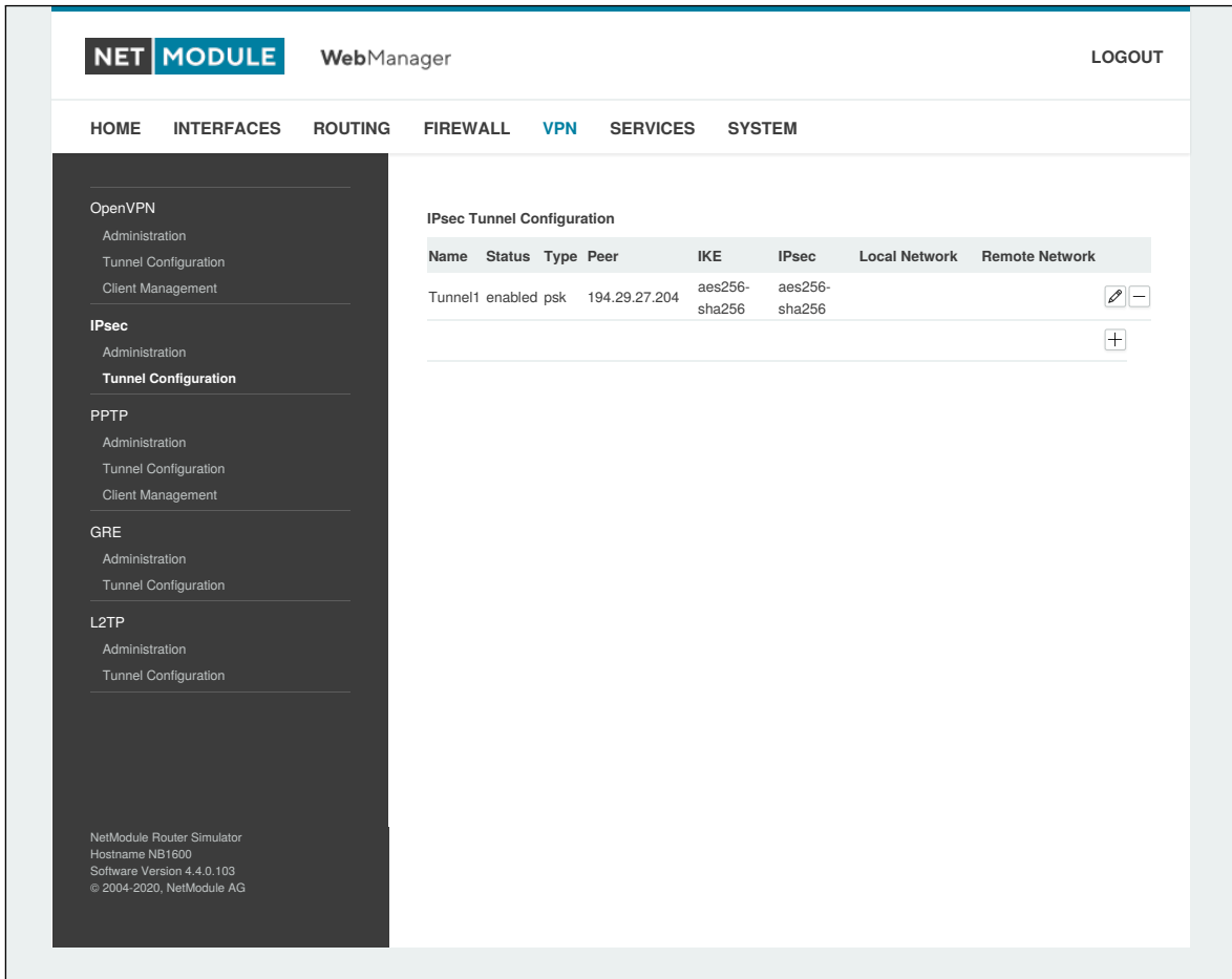
Abbildung 5.35.: IPsec-Konfiguration
