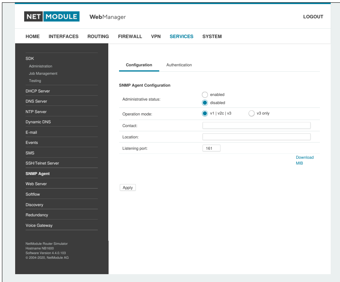
Abbildung 5.49.: SNMP-Agent
