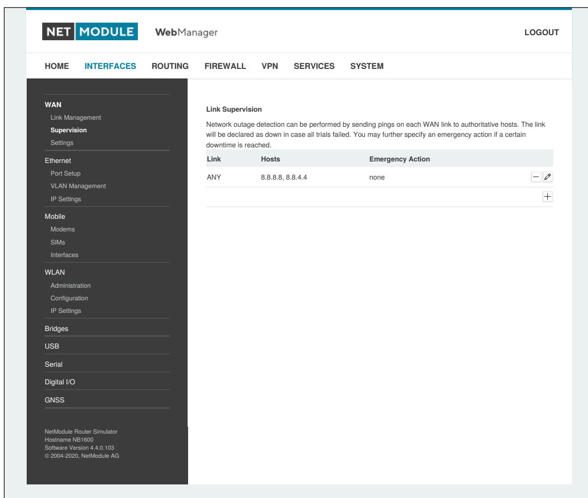
Abbildung 5.4.: Verbindungsüberwachung
