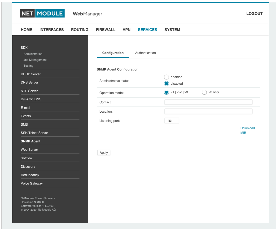
Abbildung 5.49.: SNMP-Agent
