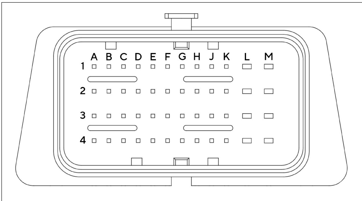
Abbildung 3.4.: X48 Outline
