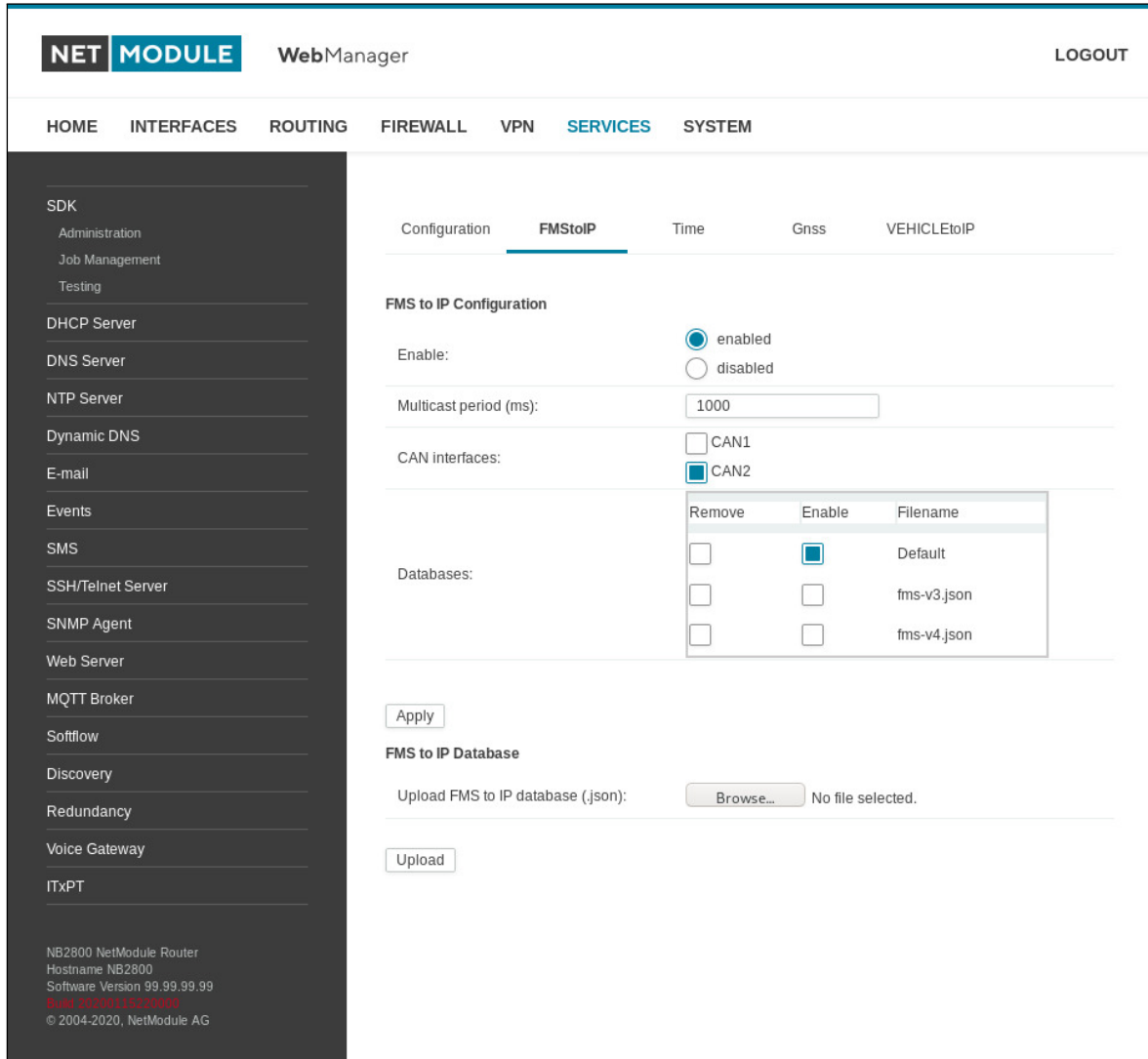
Abbildung 5.51.: ITxPT FMS-to-IP
