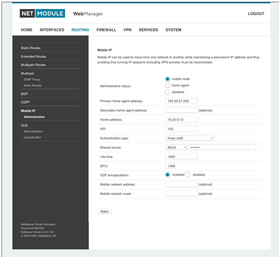
Abbildung 5.24.: Mobile IP
