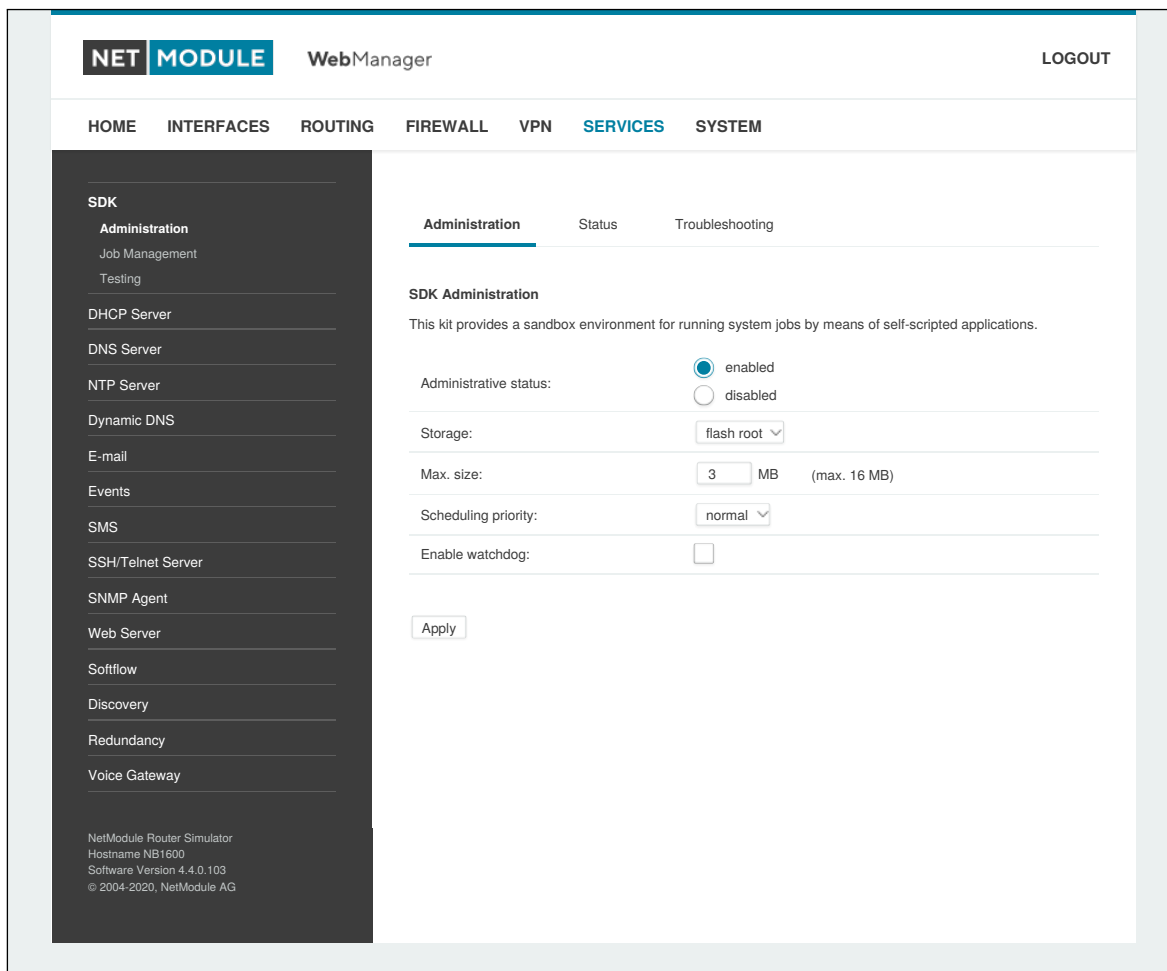
Abbildung 5.40.: SDK-Verwaltung
