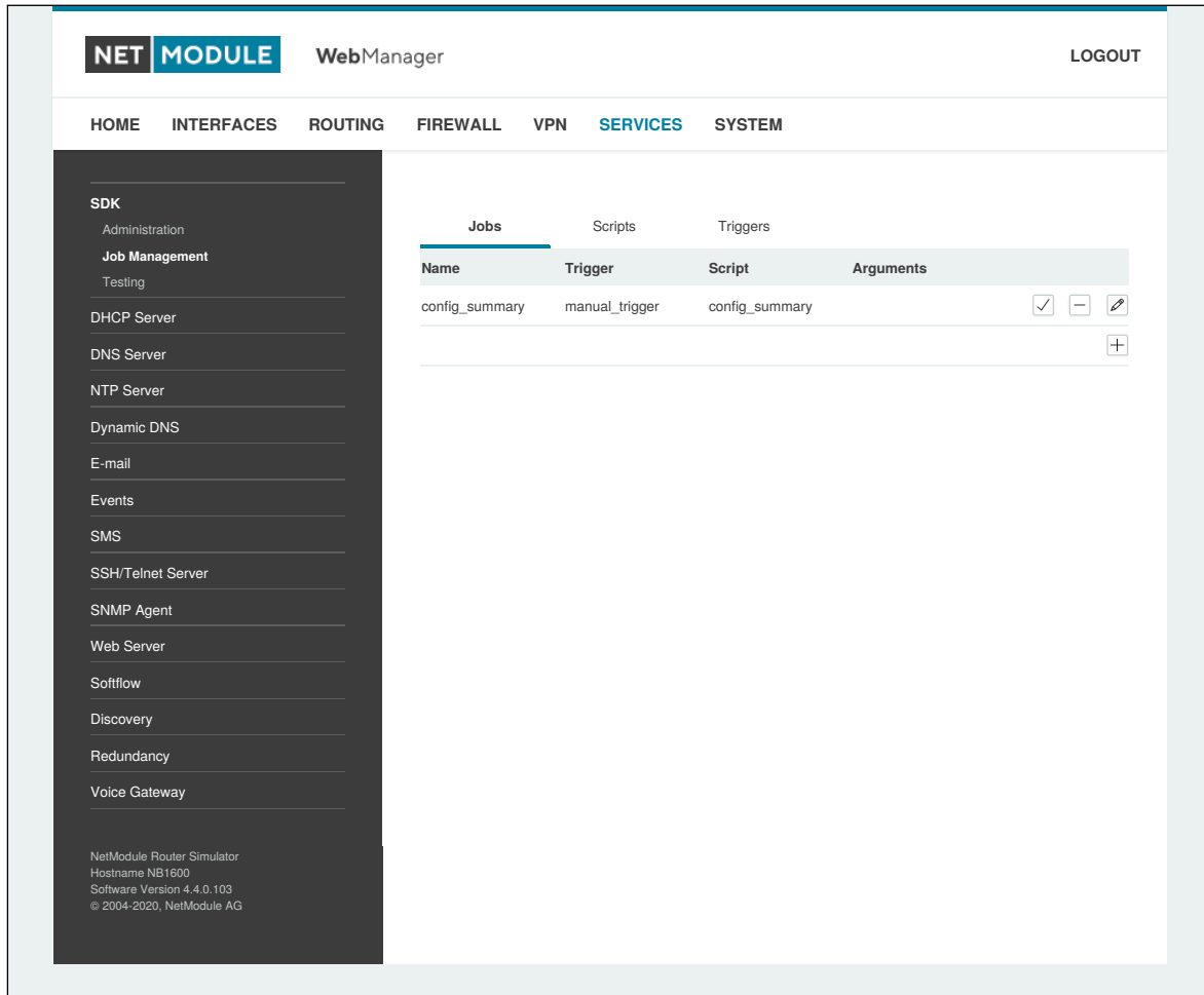
Abbildung 5.39.: SDK-Jobs
